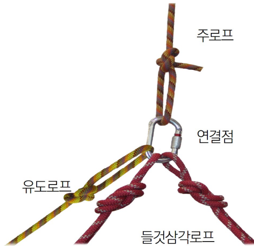
[ 그림 4-161 ] 주·보조로프와 삼각로프가 연결된 카라비너
