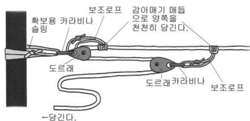
[그림 4-56] Z자형 도르래 배치법을 응용한 로프 연장법
