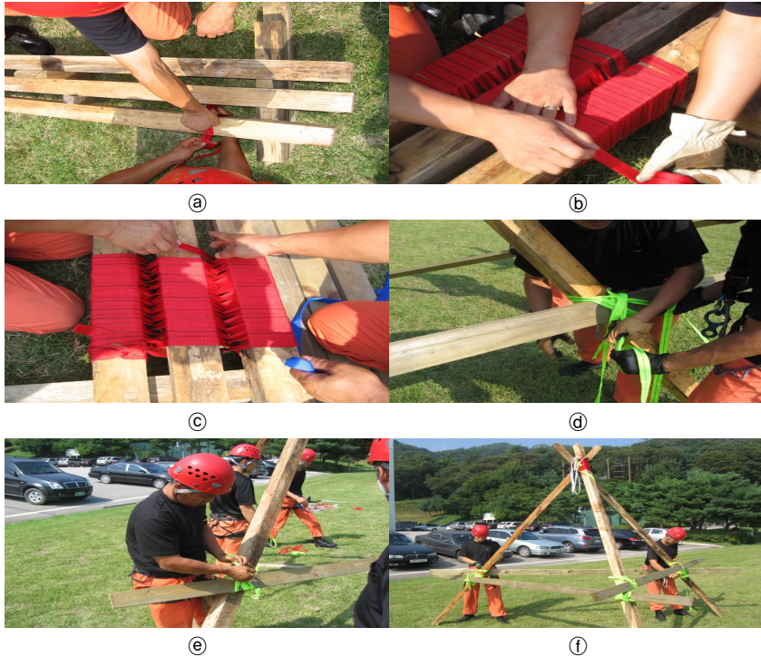
[ 그림 4-65 ] 삼각대 설치 순서
