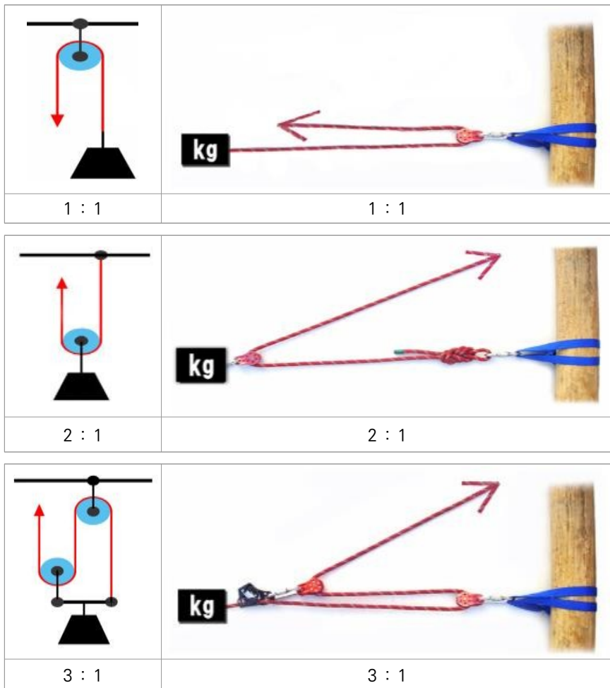
[ 그림 3-50 ] 도르래 운용방법
