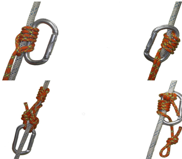
[ 그림 4-157 ] 여러 가지 방법을 응용한 감아매기
