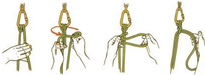
[ 그림 4-50 ] 회수 매듭법
