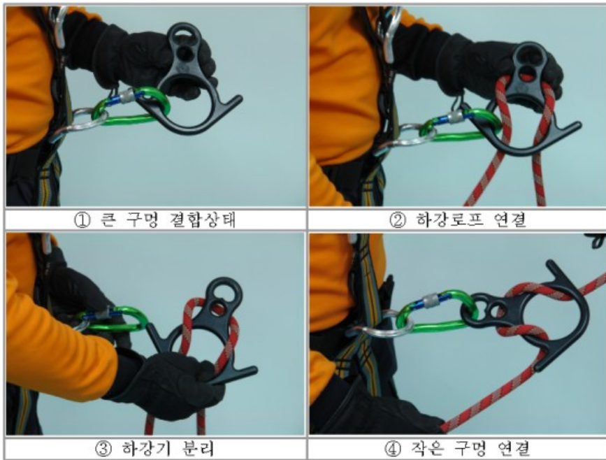
[그림 3-44] 8자하강기 올바른 사용법
