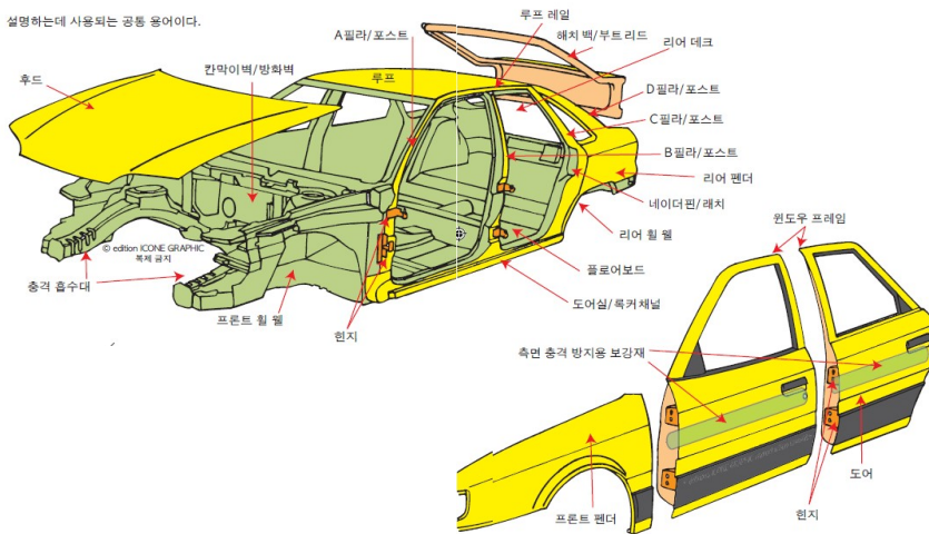
[ 그림 4-199 ] 차량의 구조 및 용어
