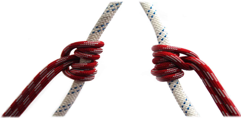
[ 그림 4-156 ] 감아매기(푸르직매듭과 클렘하이스트)
