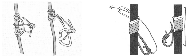
[ 그림 4-24 ] 감아매기(좌)와 클램하이스트 매듭(우)
