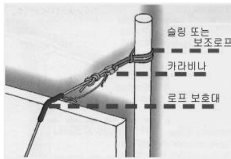
[그림 4-46] 현수로프의 간접 고정
