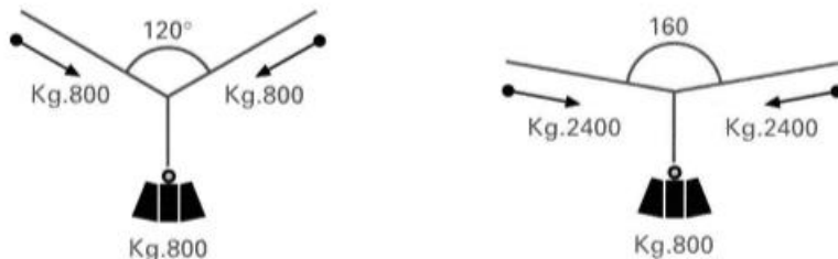
[ 그림 4-51 ] 수평으로 연장된 로프에 가해지는 장력
