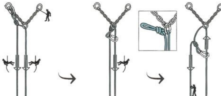
[ 그림 4-49 ] 회수로프 설치방법
