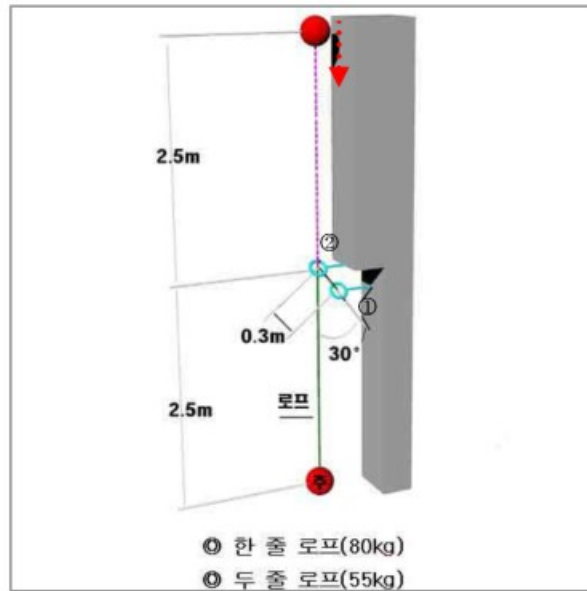
[ 그림 3-7 ] 충격흡수력 시험
