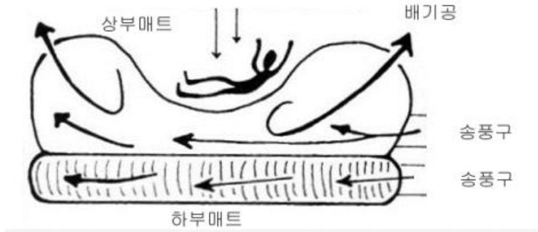
[ 그림 3-22 ] 공기매트의 구조
