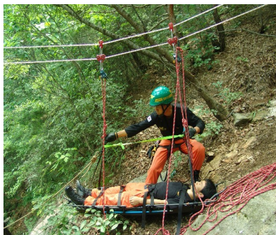
[ 그림 4-143 ] 조절장치를 이용한 요구조자 구출
