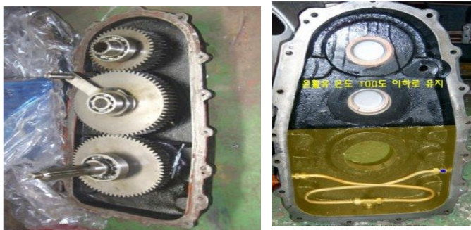
[그림 3-55] B지점, PTO내 냉각수 배관
