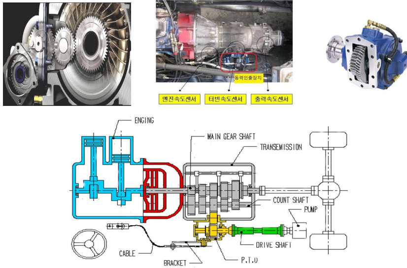
[ 그림 3-4 ] 자동변속기 P.T.O 구조
