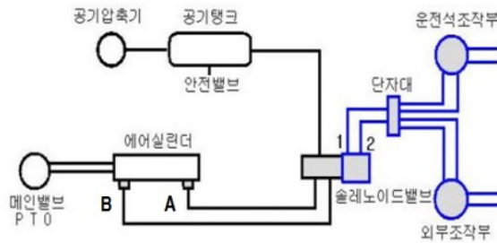
[그림 3-7] 전기식 P.T.O 작동 계통도
