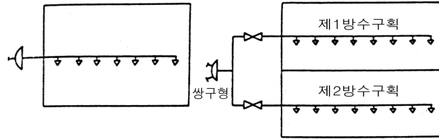
[ 그림 1-99 ] 연결살수설비 계통도
