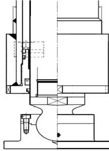
[그림 4-2] 아웃트리거 슈 및 원형 잭 실린더 구조
