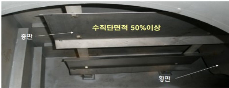
[그림 3-58] 물탱크 내부 방파판
