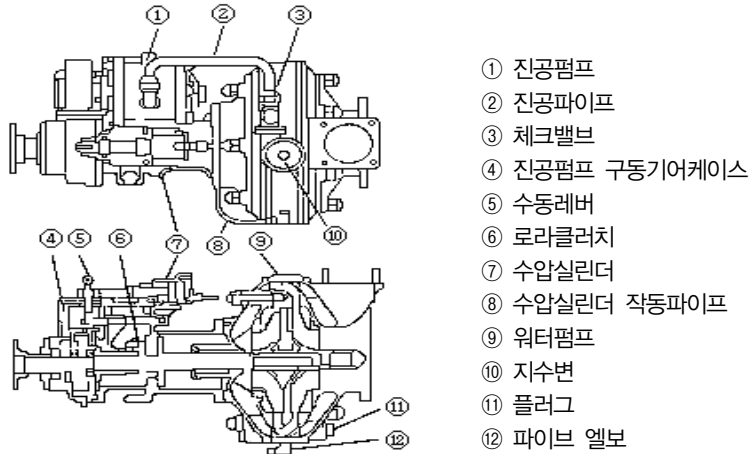
수압실린더 이용한 동력전달
