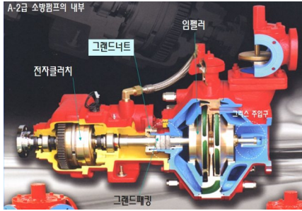
[그림 3-13] A2급 소방펌프단면도
