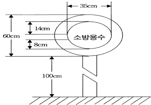
[그림 2-6] 소방용수시설 표지
