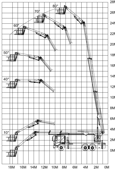
20M급 혼합 굴절사다리차
