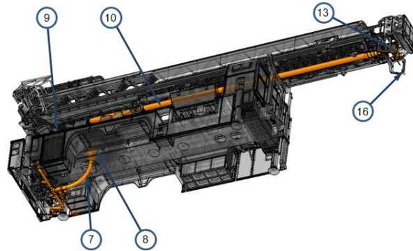
사다리차용 송수용 배관 및 방수총
