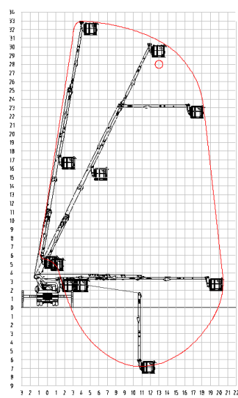
50M급 혼합 굴절사다리차
