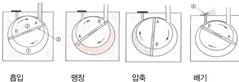
[그림 3-24] 진공펌프 원리
