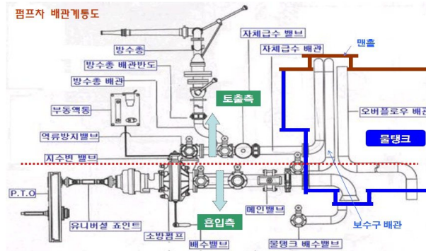
[ 그림 3-12 ] 소방자동차 배관계통도 및 펌프주변 장치
