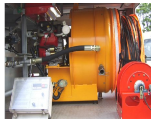
고발포 장치
