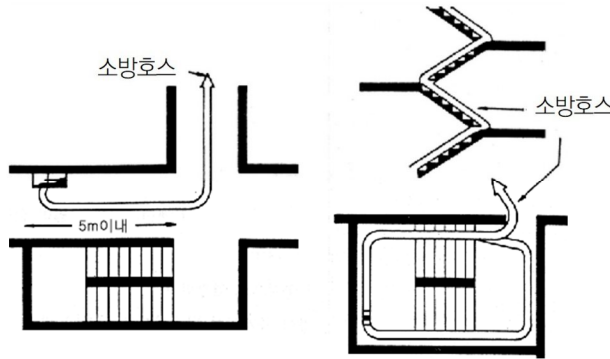
[ 그림 1-63 ] 연결송수관 사용의 경우
