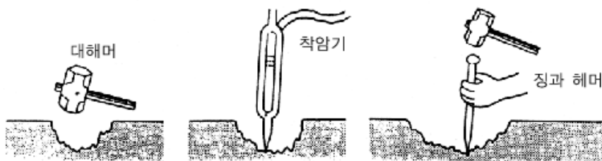
[그림 1-90] 바닥 파괴 요령
