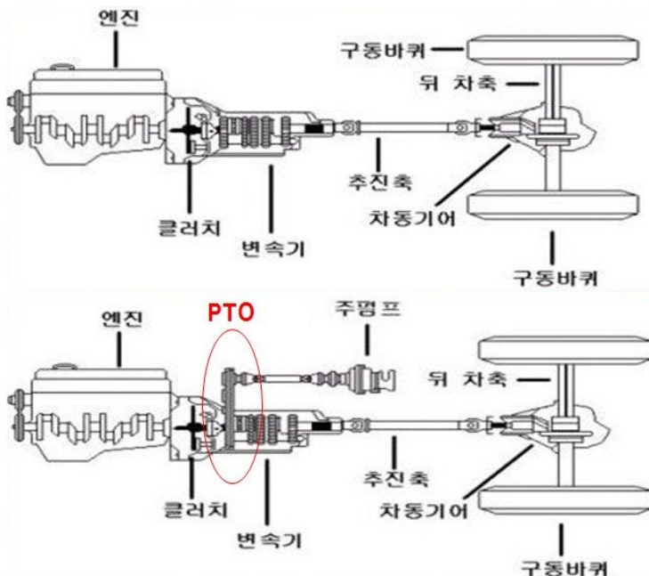
[그림 3-1] P.T.O 장착 전·후 비교
