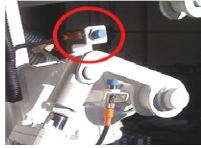
사다리 록킹 열림 센서 사다리 록킹 닫힘 센서
