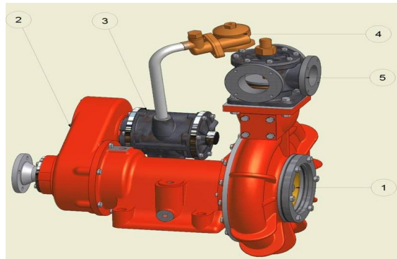
[그림 3-15] A1급 소방펌프 주변장치
