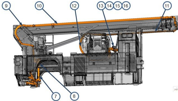
굴절차용 송수용 배관 및 방수층
