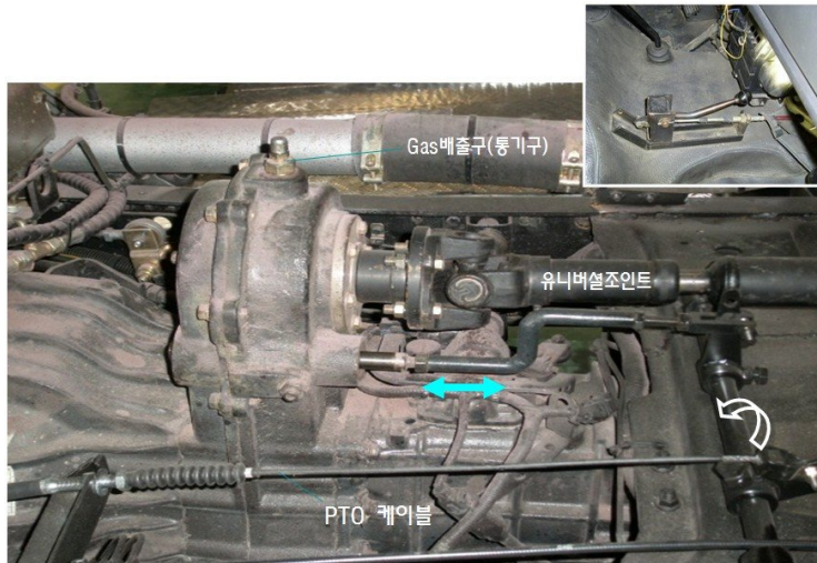
[그림 3-6] P.T.O 작동 케이블방식
