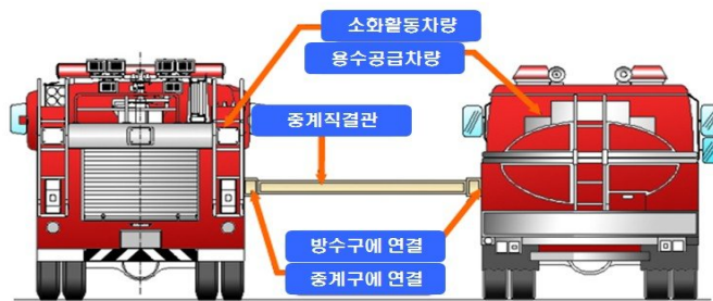
[ 그림 3-44 ] 중계관을 이용한 급수
