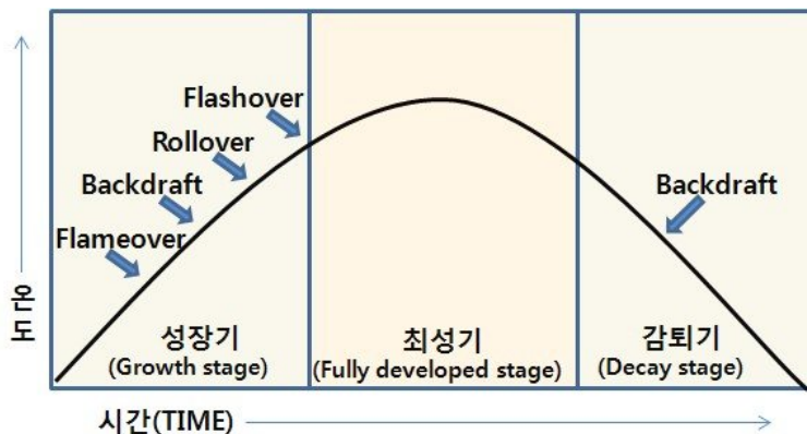
[그림 1-6] 시간과 온도변화에 따른 연소 이상현상
