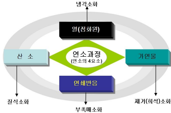
[ 그림 1-11 ] 연소의 4요소와 소화원리
