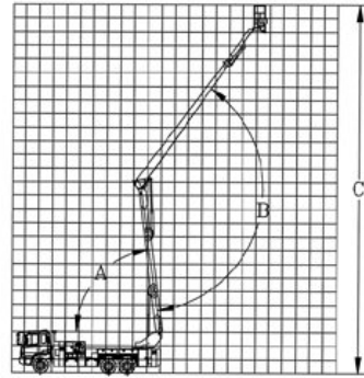
27M급 굴절식 사다리(남영)
