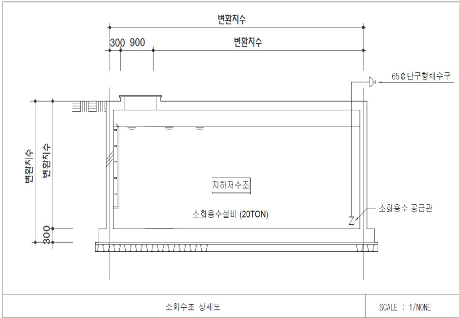
[그림 2-7] 저수조 구조도
