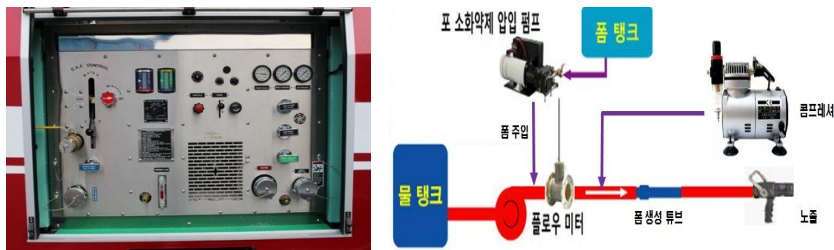
[그림 3-73] CAFS 방식
