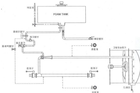
고발포 구성도
