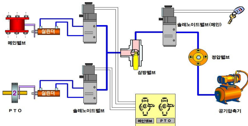
[ 그림 3-8 ] 에어컨트롤장치 계통 이해도
