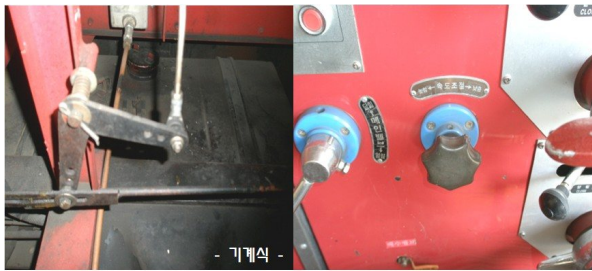
[ 그림 3-39 ] 기계식
