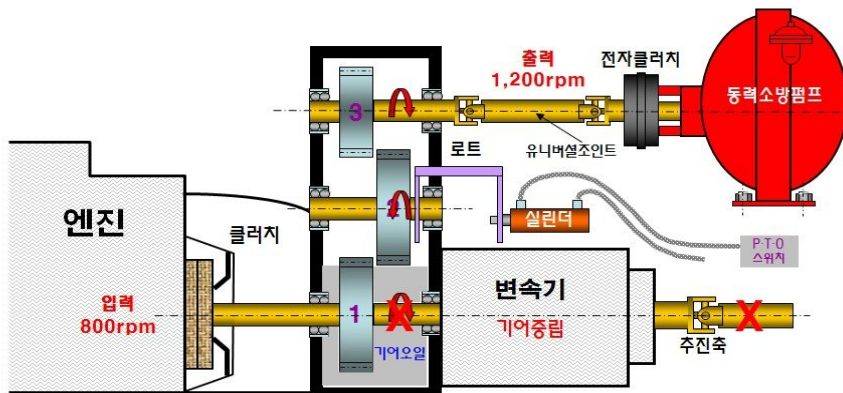
[그림 3-3] P.T.O 내부 구조 이해도
