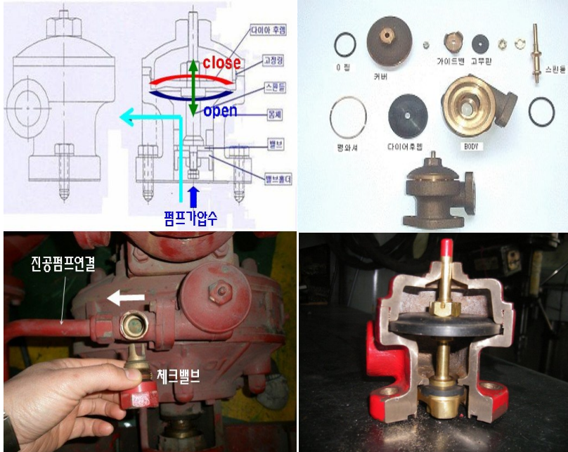
[ 그림 3-36 ] 지수밸브의 구조
