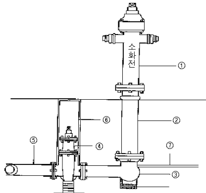
[그림 2-3] 지상식 소화전 구조도
