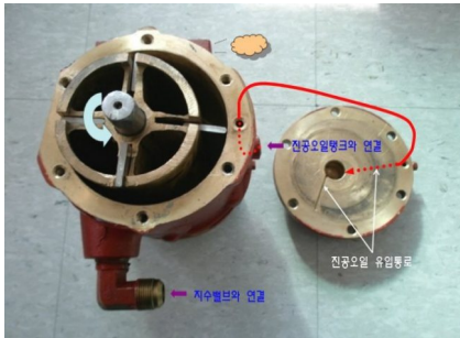
[그림 3-29] 진공오일 급유흐름도
