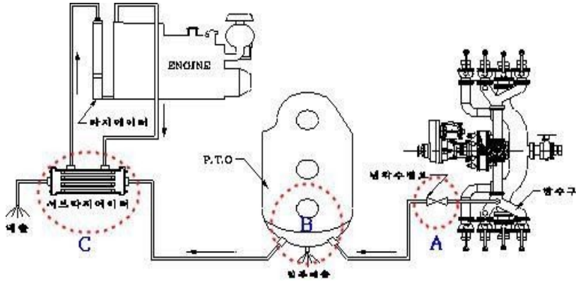
[그림 3-53] PTO 냉각라인 계통도
