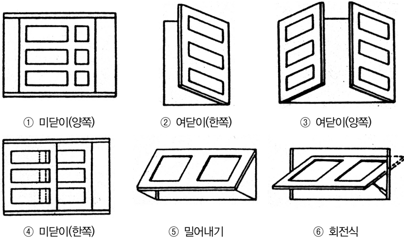
[ 그림 1-22 ] 창의 개방방식구분
