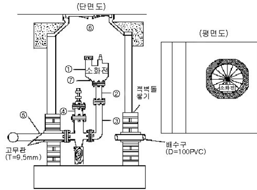
[그림 2-2] 지하식 소화전 구조도
