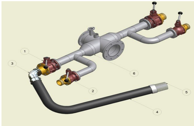
[ 그림 3-41 ] 흡수배관도
