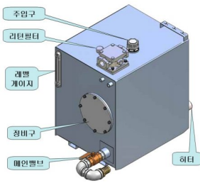
유압유 탱크
