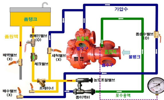
[ 그림 3-70 ] 펌프 프로포셔너 방식
