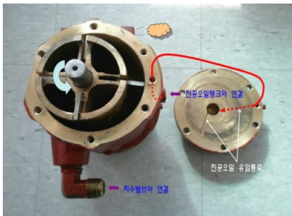
[ 그림 3-32 ] 진공오일 급유흐름도
