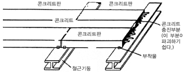
[ 그림 1-92 ] PC 콘크리트판의 바닥구조
