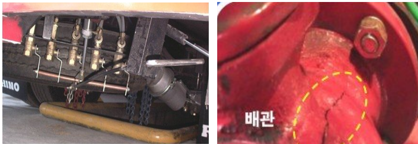
[ 그림 3-52 ] 자동배수밸브 및 배수불량으로 배관 동파
