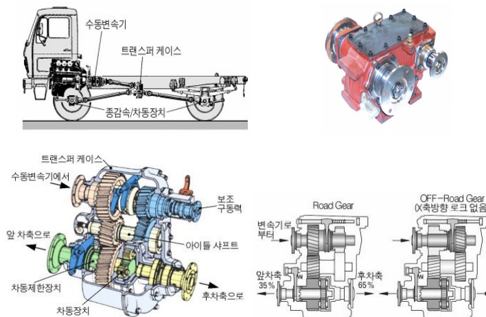
[ 그림 3-5 ] 복합 P.T.O 구조
