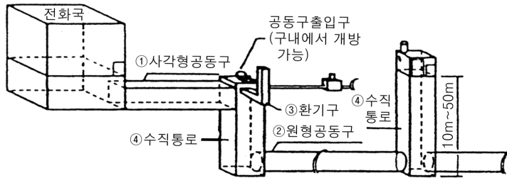
[그림 1-133] 공동구 계통도
