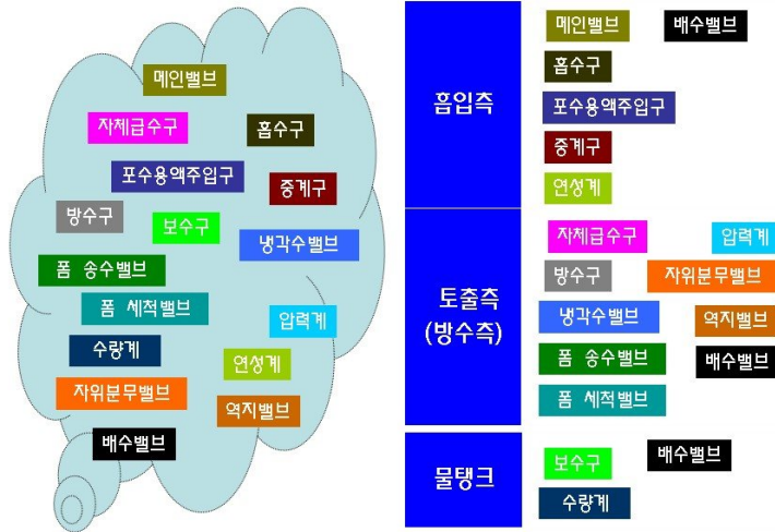
[그림 3-66] 펌프기준 배관 및 밸브 등의 위치
