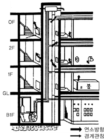
[ 그림 1-78 ] 파이프샤프트에 대한 관창배치
