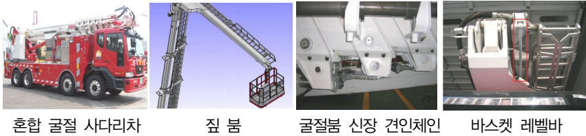
혼합 굴절 사다리차 짐 붐 굴절붐 신장 견인체인 바스켓 레벨바
