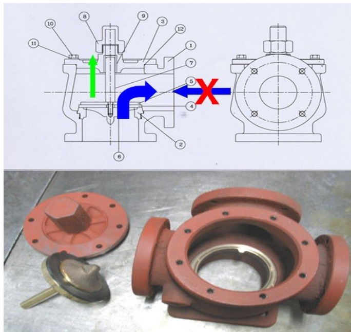
[ 그림 3-37 ] 역류방지밸브의 구조
