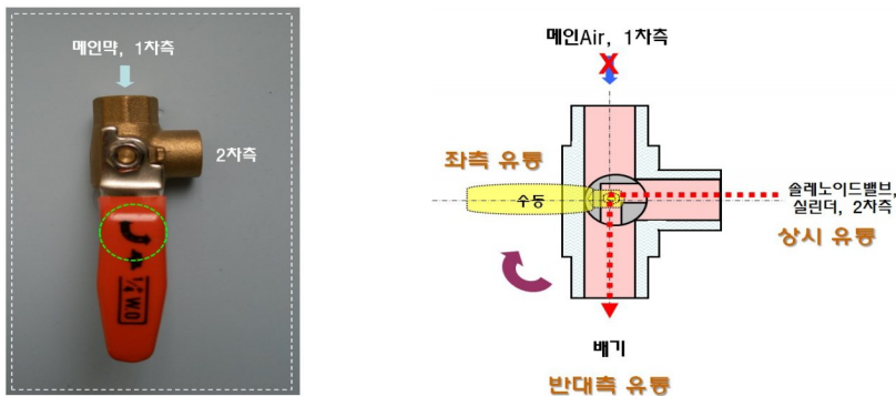
[그림 3-10] 솔레노이드밸브 및 수동전환밸브
