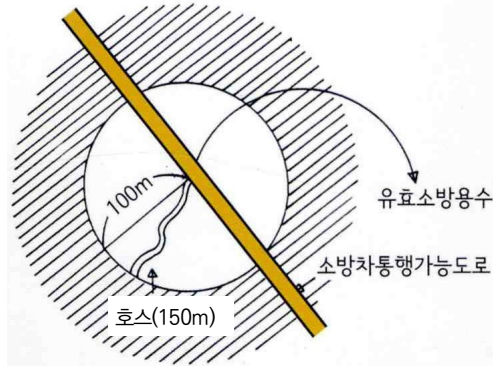
[그림 1-12] 소방호스 연장과 도달거리의 관계
