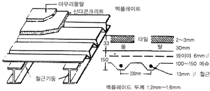
[ 그림 1-91 ] 텍플레이트조 바닥의 구조
