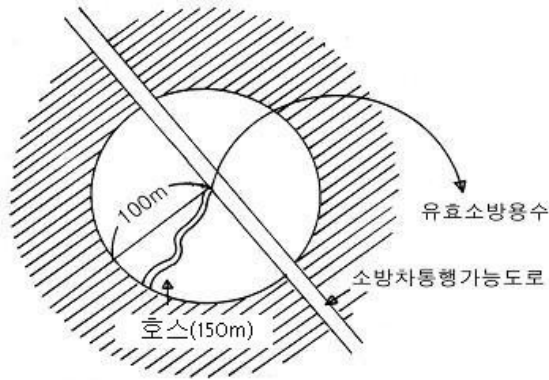
[그림 2-1] 소방호스 연장과 도달거리의 관계
