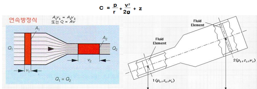
[ 그림 3-68 ] 베르누이 정리
