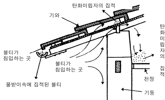
[ 그림 1-107 ] 처마 속으로 침입하는 불티와 탄화물의 집적장소
