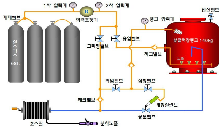
[ 그림 3-75 ] 분말장치 구성도
