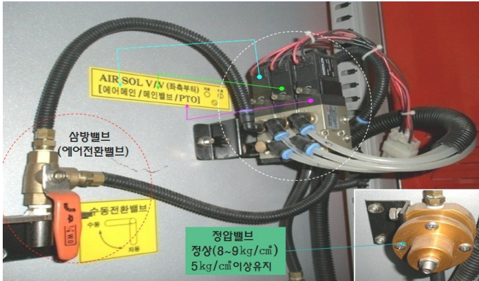
[그림 3-9] 솔레노이드밸브 및 수동전환밸브
