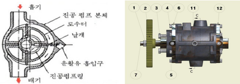
[그림 3-23] 진공펌프내부 및 외관도
