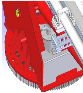
스위블 조인트
