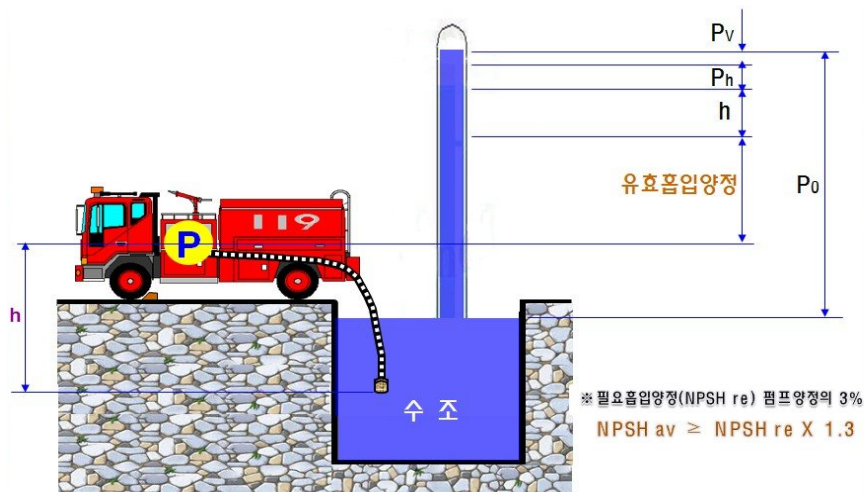
[ 그림 3-80 ] NPSH av 유효흡입양정
