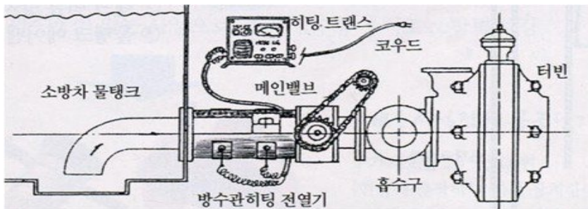
[ 그림 3-51 ] 히팅장치
