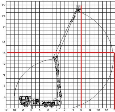
27M급 굴절식 사다리(남영)
