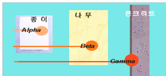
[ 그림 1-131 ] 방사선별 투과력의 비교
