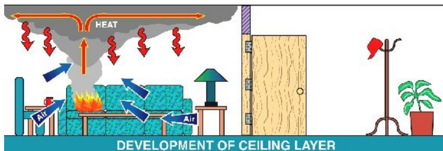
[그림 1-4] 구획실내의 온도 상승
