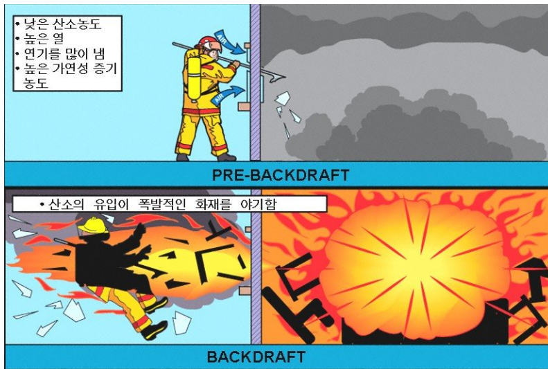
[그림 1-7] 백드래프트 현상
