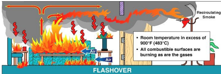
[그림 1-9] 플래쉬오버
