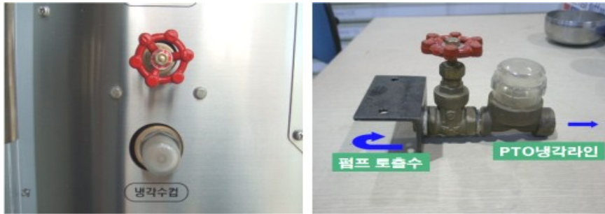
[그림 3-54] A지점, 냉각수 밸브 및 스트레이너
