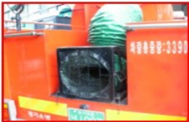
4) 흡입구를 원하는 장소에 배치한다.
