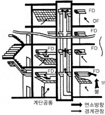
[ 그림 1-79 ] 닥트 부분에 대한 관창 배치
