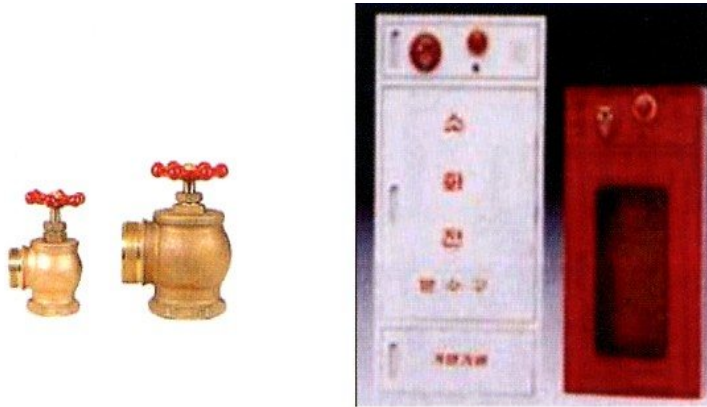
[그림 7-2] 옥내소화전 방수구 및 소화전함
