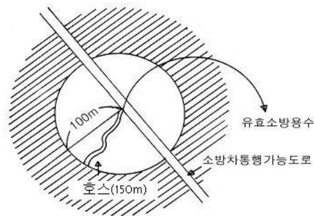
소방호스 연장과 도달거리의 관계
