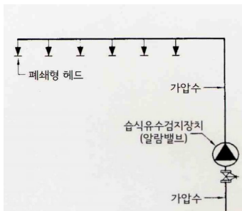
습식(Wet pipe system)
