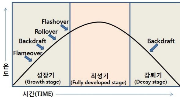
[ 그림 3-3 ] 시간과 온도변화에 따른 연소 이상현상
