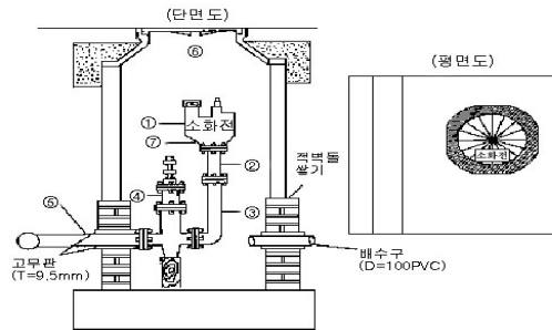
[ 그림 8-1 ] 지하식 소화전 구조도
