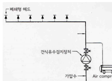
건식(Dry pipe system)
