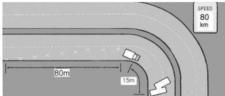
[ 그림 4-173 ] 곡선도로 사고발생 시 유도표지
