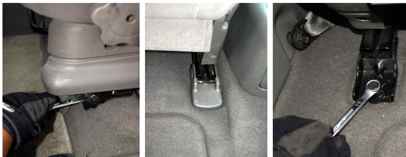
[ 그림 4-192 ] 운전석 의자를 분리하는 방법
