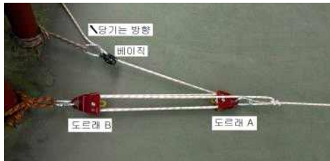
[ 그림 4-57 ] 2단도르래를 이용한 로프 연장 방법
