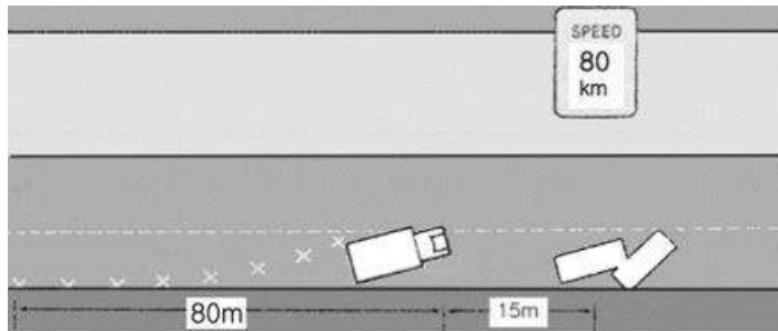
[ 그림 4-172 ] 자동차 사고 시 유도표지 설치
