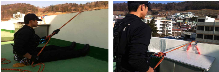
[ 그림 4-72 ] 신체에 직접 결착한 간접하강
