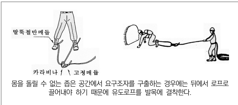
[그림 4-35] 폐쇄공간에서 요구조자 구출방법
