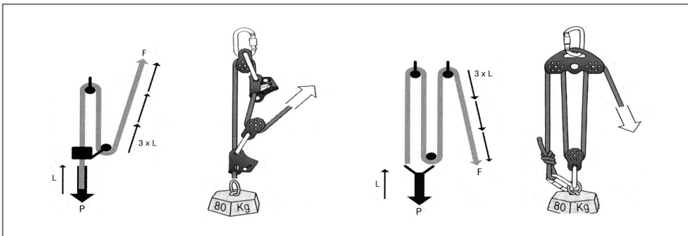
[그림 2-12] 도르래 설치방법의 예
