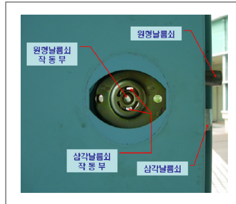
[그림 6-2] 방화문 잠금장치(내부)
