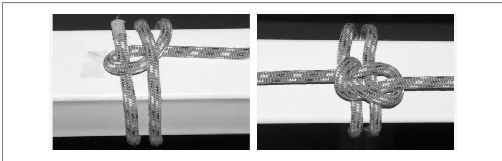
[그림 3-23] 잡아매기
