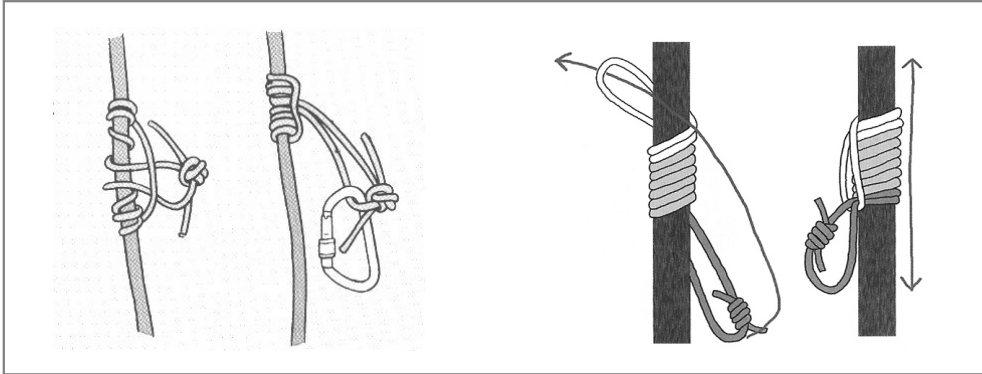
[그림 3-24] 감아매기(좌)와 클렘하이스트 매듭(우)
