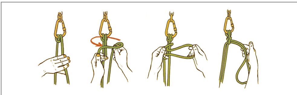
[그림 3-54] blocking loop
