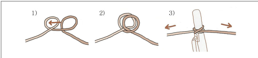
[그림 3-20] 말뚝매기의 다른 방법, 로프 끝을 둥글게 겹쳐서 끼운다.
