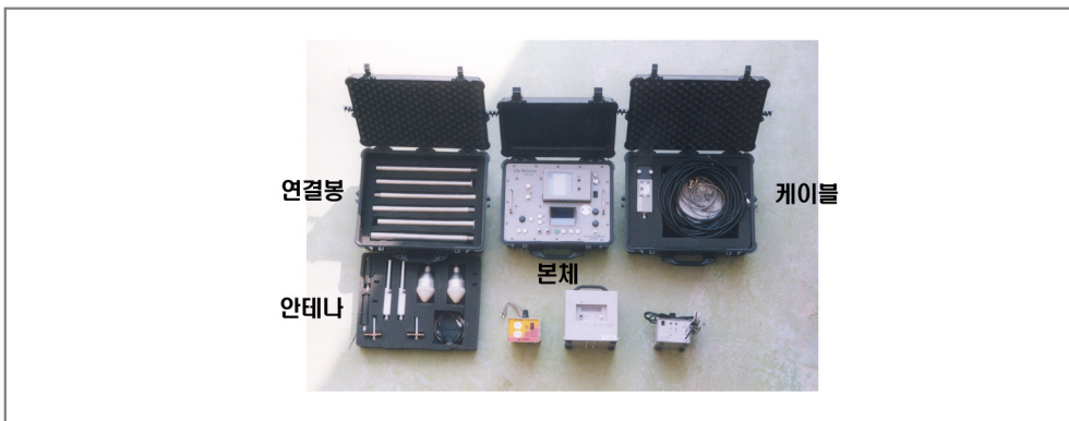
[그림 2-25] 매몰자전파탐지기
