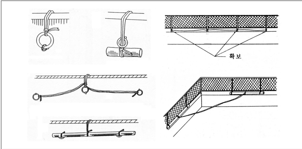
[그림 3-45] 옥상의 설치물을 이용하기 [그림 3-46] 펜스를 이용하는 방법
