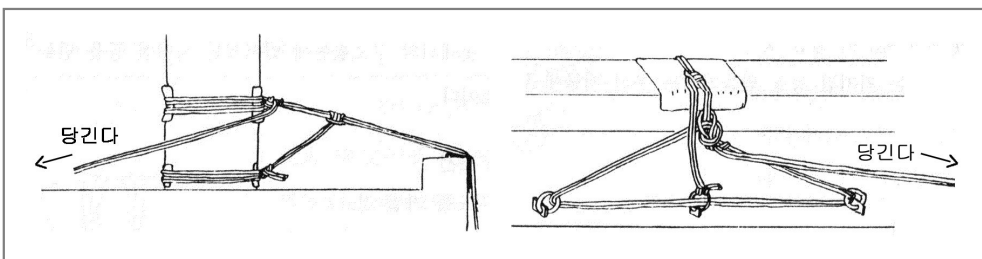
[그림 3-44] 기둥과 난간의 활용방법
