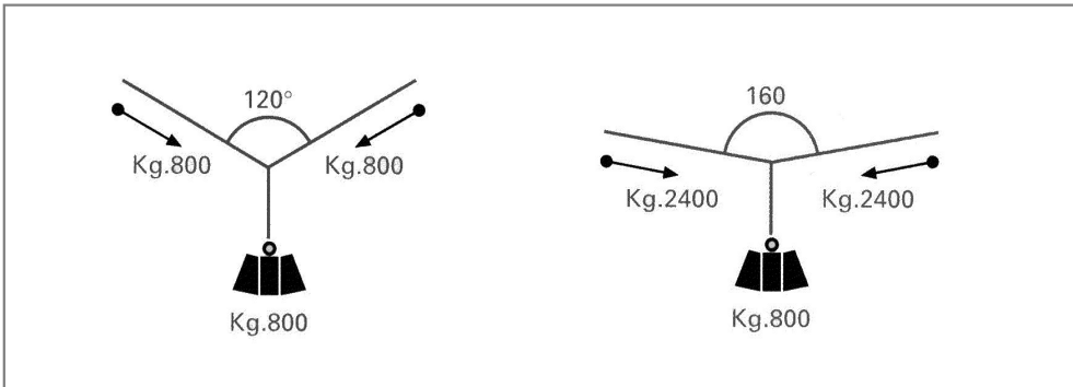
[그림 3-55] 수평으로 연장된 로프에 가해지는 장력
