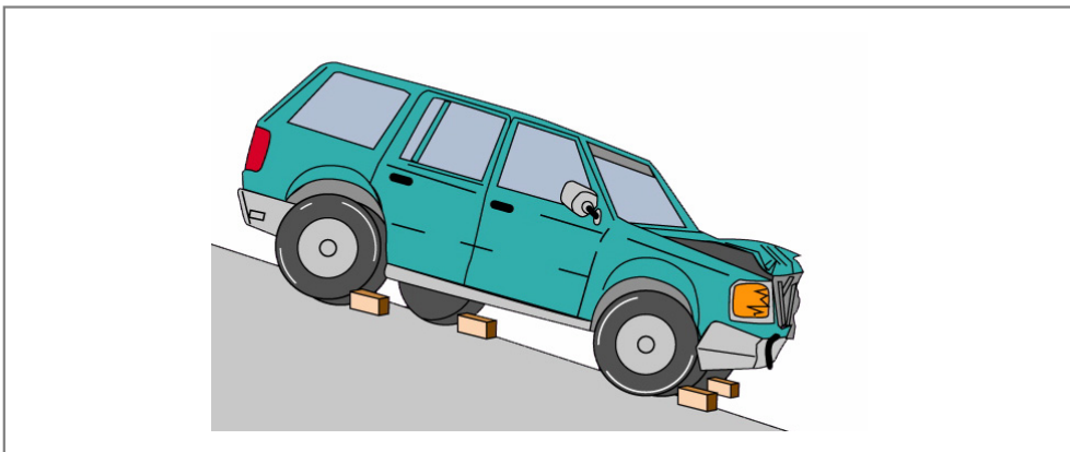
[그림 5-18] 차체에 고임목을 대는 방법
