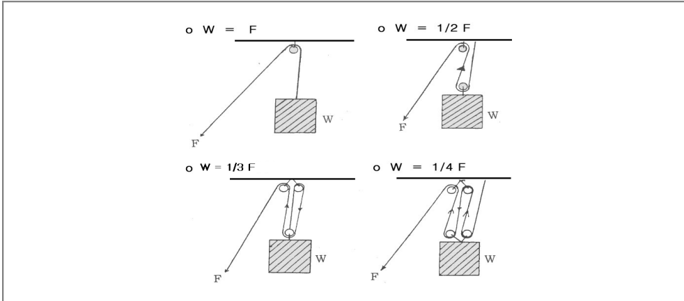
[그림 2-11] 도르래 숫자와 힘의 이득 관계
