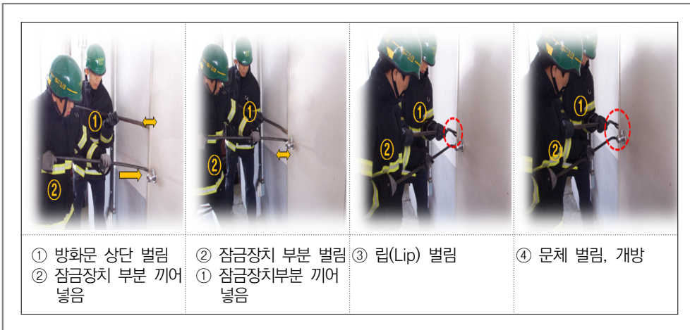
[그림 6-26] 해정공구
