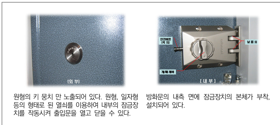
[그림 6-3] 보조 잠금장치
