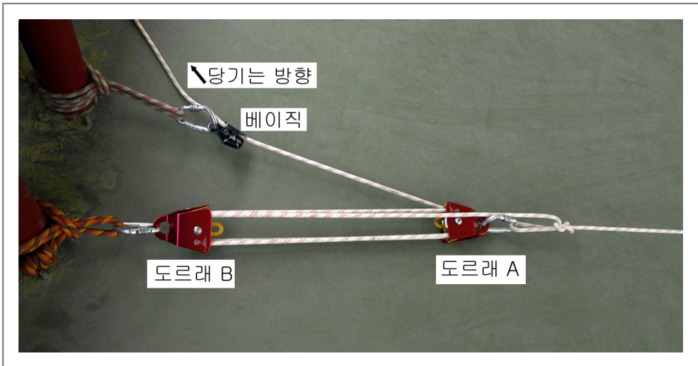
[그림 3-61] 2단 도르래를 이용한 로프 연장 방법
