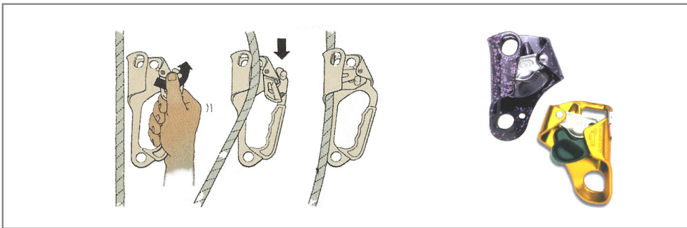
[그림 2-9] 등강기를 로프에 삽입하는 방법 [그림 2-10] 베이직(상), 크롤(하)
