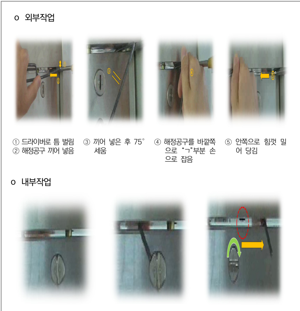
[그림 6-27] 유리출입문 강제개방
