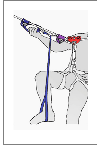
[그림 3-97] 도하장비 결착
