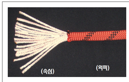
[그림 2-2] 컨먼틀 로프의 구조
