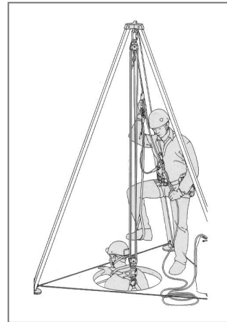
[그림 2-20] 맨홀 구조기구
