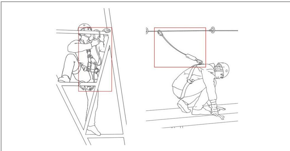
[그림 3-65] 자기확보 취하기
