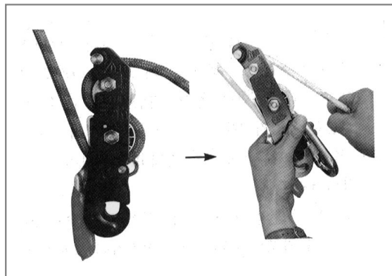
[그림 2-7] 스톱 하강기 사용법
