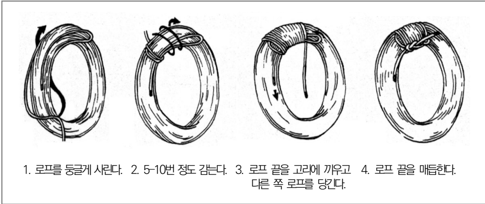
[그림 3-31] 둥글게 사리기
