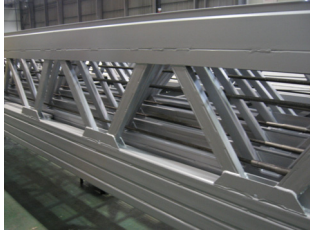
사다리 구조물(측면)
