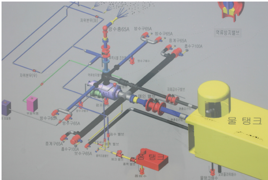
소방펌프 배관 계통도
