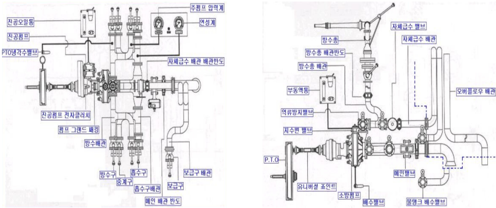
소방펌프 배관 계통도
