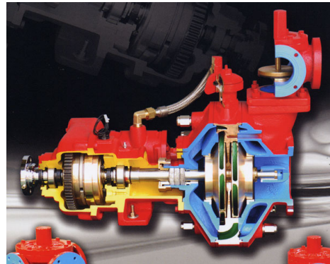
소방펌프 입체도
