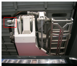
혼합 굴절식 짐 붐 각도 센서
