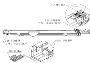
체인롤러 & 케이블베어
