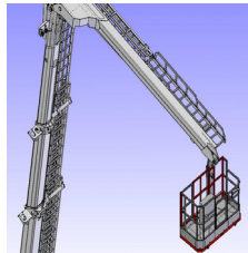
혼합굴절식사다리장착모습 혼합굴절식짐붐단면도 혼합 굴절식붐신장견인체인 바스켓 레벨바
