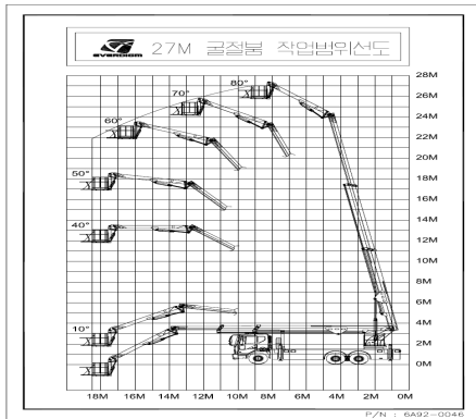
27M급 혼합 굴절식 사다리차
