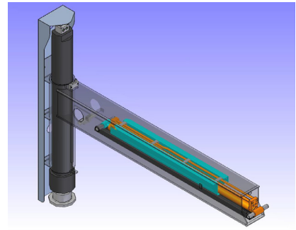
원형 아웃트리거 실린더 조립상태
