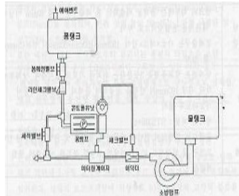
프레셔사이드 프로포셔닝방식
