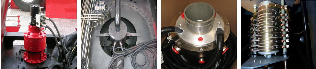
감속기 실제사진 스위블 조인트 장착상태 스위블 조인트 단품상태 스위블 조인트 내부
