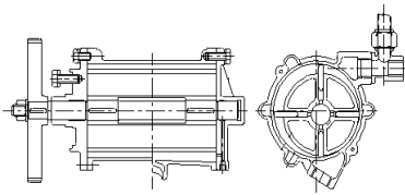
진공펌프 단면도
