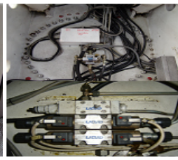
승강기 수동 솔레노이드밸브
