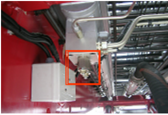
직진식 신장 · 수축 확장 실린더 카운터 밸런스 밸브
