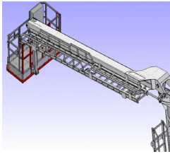
혼합굴절식짚뿔및 바스켓(에버다임)
