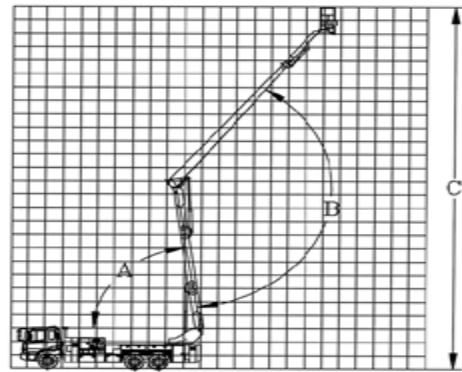
27M급 굴절식 사다리(남영)
