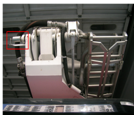
짚 붐 각도 센서
