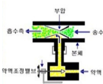
펌프 프로포셔너 방식
