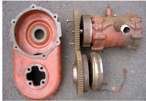
진공펌프 구동장치
