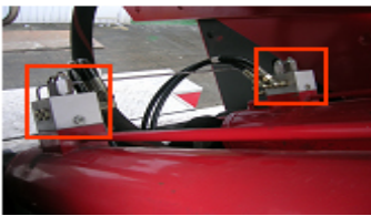
직진식 기복 상승 · 하강 확장 실린더 밸런스 밸브
