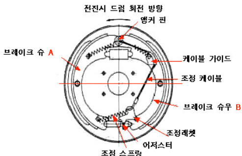
드럼 계통도
