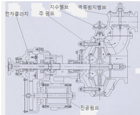
소방펌프 계통도
