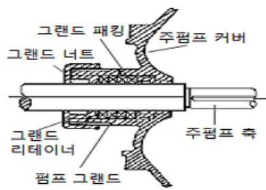
그랜드너트 단면도
