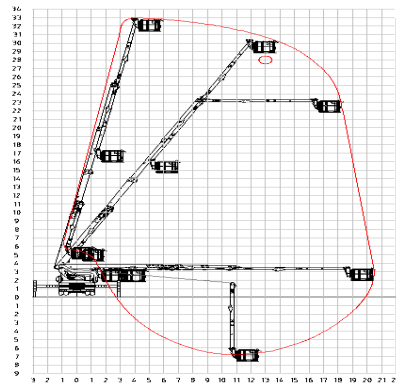
33M급 혼합 굴절식 사다리차
