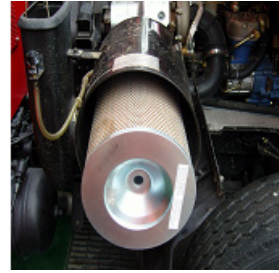
엘리먼트 탈착
