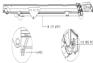
붐 신장 실린더
