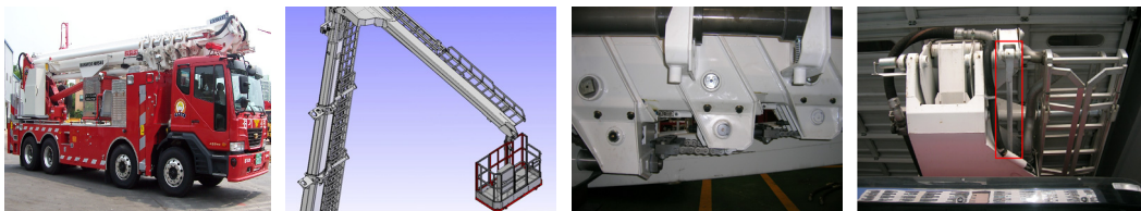
혼합 굴절 사다리 짐 붐 단면도 혼합 굴절붐신장견인체인 바스켓레벨바(혼합굴절)
