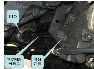
유압 메인 펌프
