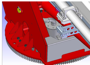
스위블 조인트 조립상태
