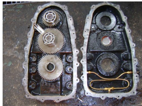
PTO 내부 모습
