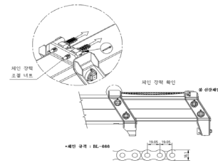
리프체인
