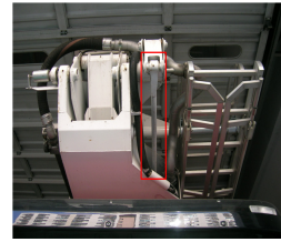
혼합굴절식바스켓 레벨바(에버다임)
