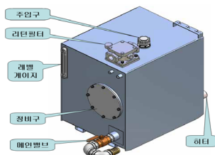
유압탱크
