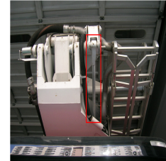
혼합굴절식사다리장착모습 혼합굴절식짐붐단면도 혼합 굴절식붐신장견인체인 바스켓 레벨바
