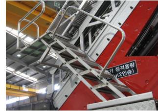
직진식 사다리 보조계단
