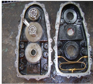
P.T.O 내부모습
