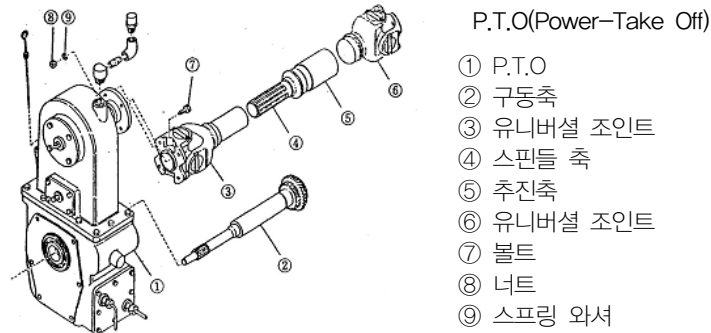
소방펌프 동력전달장치(P.T.O)의 구성 요소
