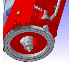
스윙기어 및 선회장치
