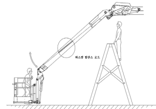
짐 붐
