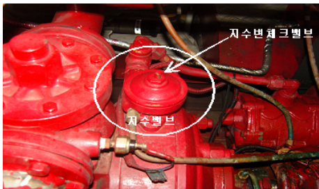
펌프 상부 부착 모습
