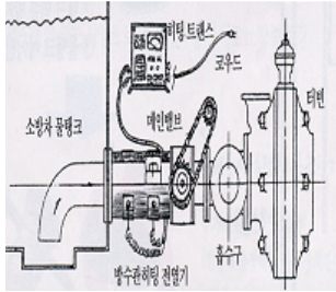
펌프배관 히팅장치 단면도
