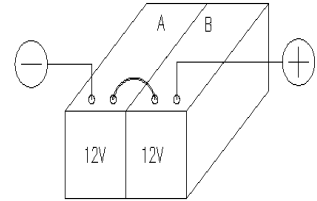
배터리 충전(점프)
