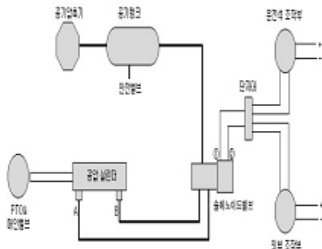
자동밸브 계통도
