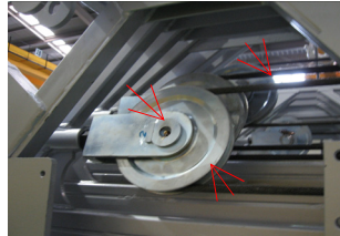
와이어 및 와이어 풀리
