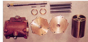
진공펌프 분해
