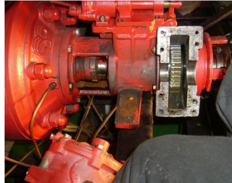
진공펌프 탈착후
