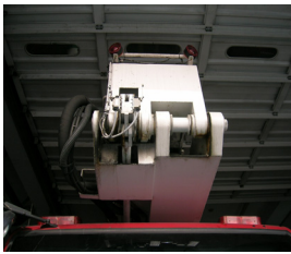
굴절식2단계복각도센서 (남영)
