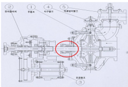
그랜드너트 위치
