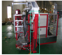
혼합 굴절식 바스켓 수평 실린더(에버다임)
