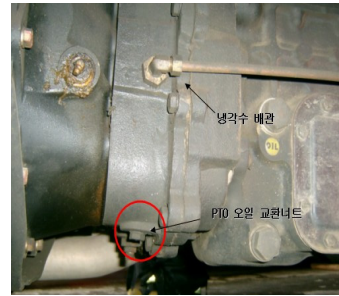
P.T.O 하부 모습
