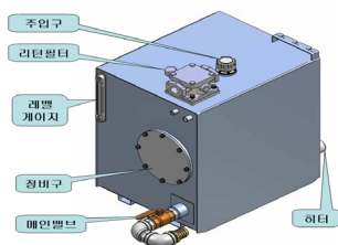
유압유 탱크
