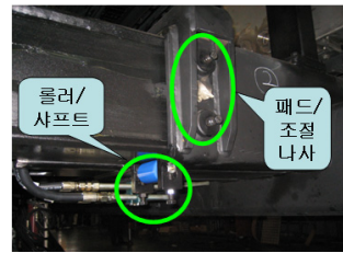
아웃트리거 롤러 및 패드
