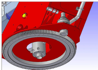
선회장치 조립
