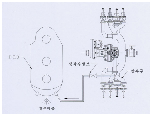
PTO 냉각장치 계통도
