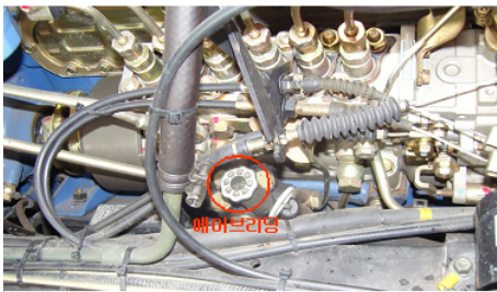
우측으로 돌리면 에어브리딩이 위로 올라온다. 에어를 제거하기위해 펌프질을 한다. 에어가 제거되고 기름이 흘러 나올때까지 열심히 펌프질...
