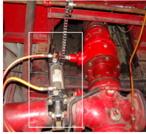
에어실린더
