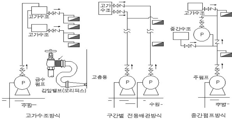
(그림 3-21) 감압방식
