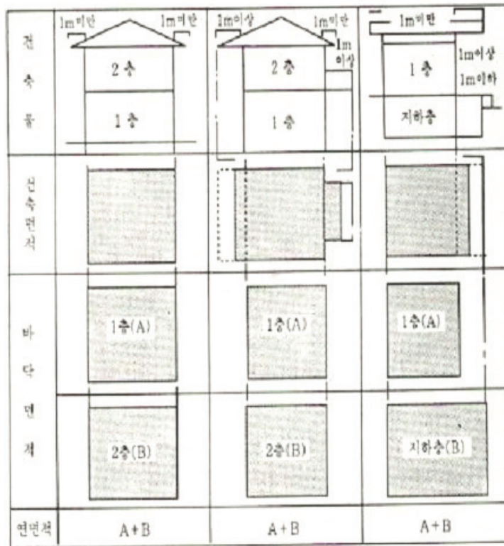
(그림 12) 면적 산정방법 예시
