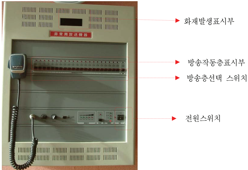
[그림 3] 비상방송설비의 스위치 및 표시등
