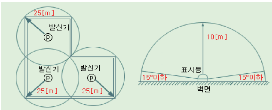
[그림39] 발신기의 설치거리
