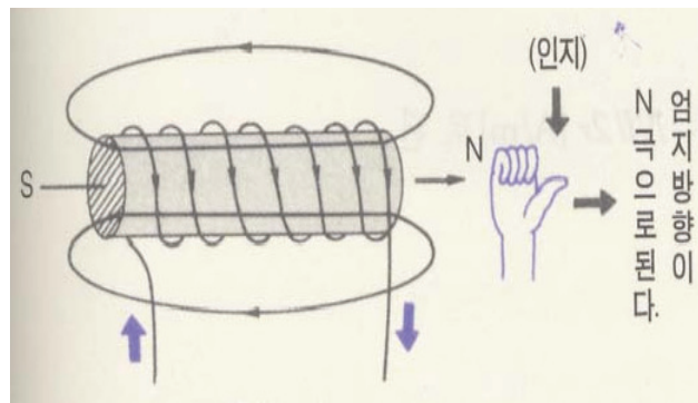
[그림 5] 전자석의 원리
