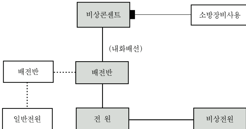
[그림 1] 비상콘센트설비의 구성
