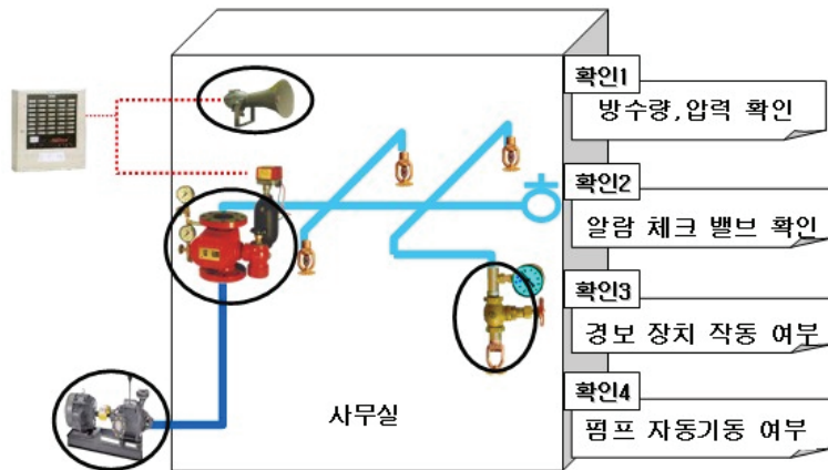
(그림 4-23) 습식스프링클러 점검사항
