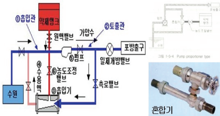
(그림 5-7) 펌프프로포셔너 방식
