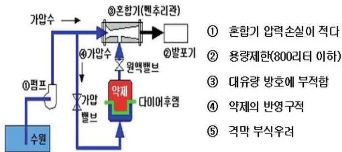
[그림 5-8] 격막이 있는 방식
