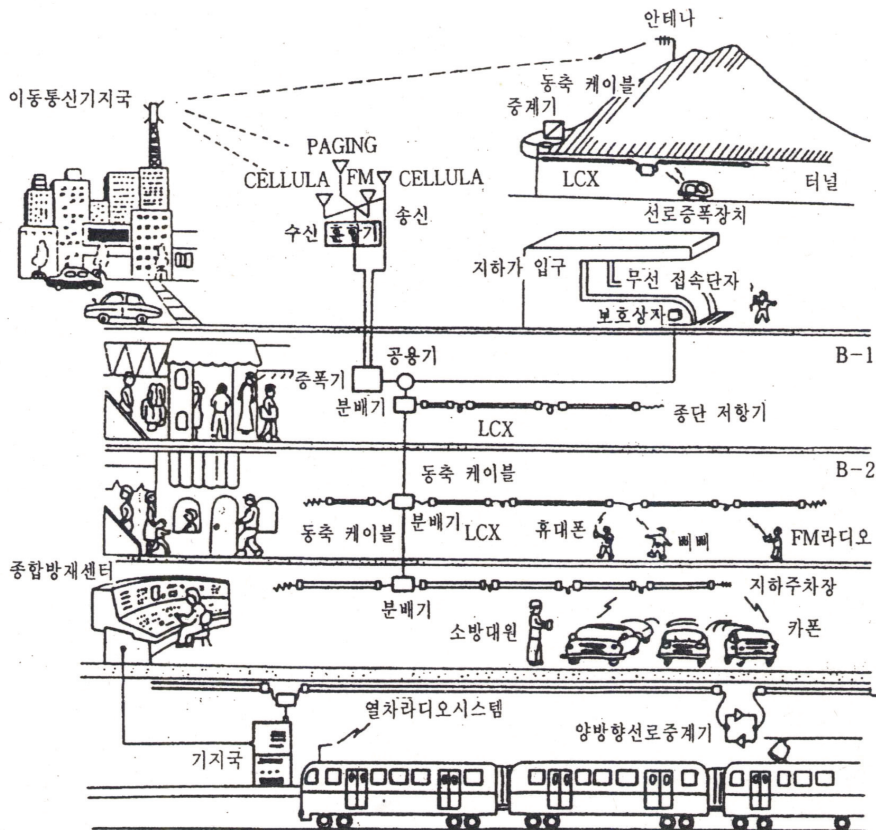
[그림 1] 무선통신보조설비의 사용
