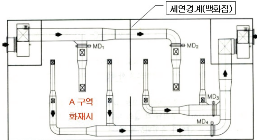
[그림 7-2] 인접구역 상호제연방식
