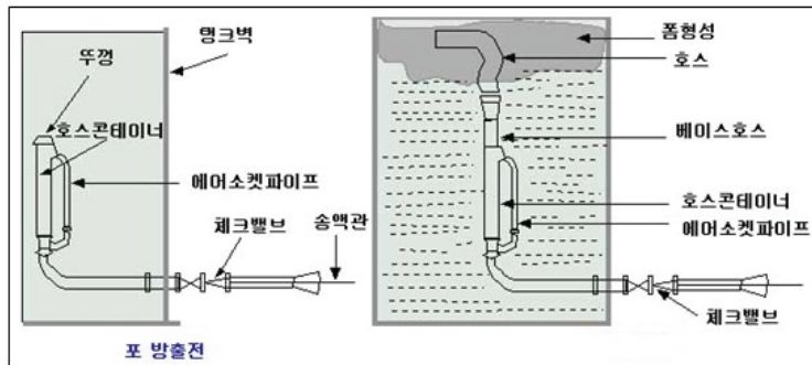
(그림 5-18) 반표면하 방식
