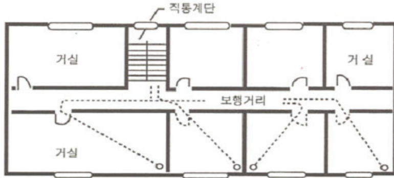
[그림 28] 직통계단까지 보행거리
