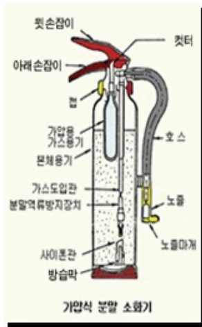
(그림 2-8) 가압식 분말소화기 점검
