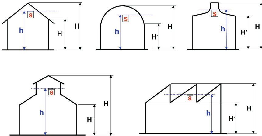
[그림 31] 건축물별 감지기의 설치높이 산정방법
