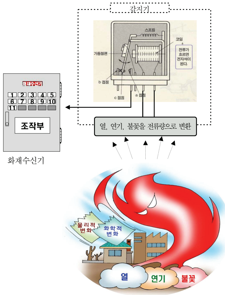
(그림 6) 전자석을 이용한 점점구성 방법
