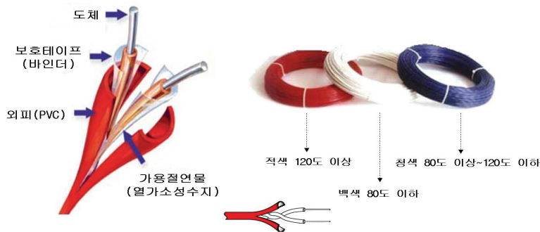
(그림 16) 정온식감지선형감지기의 형태 및 표시
