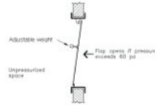
플랩댐퍼 방식 (FLAP DAMPER)
