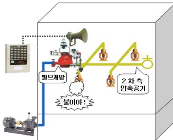
[그림 4-9] 건식스프링클러설비 구성
