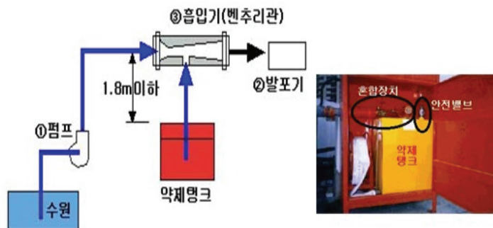
(그림 5-6) 라인프로포셔너 방식
