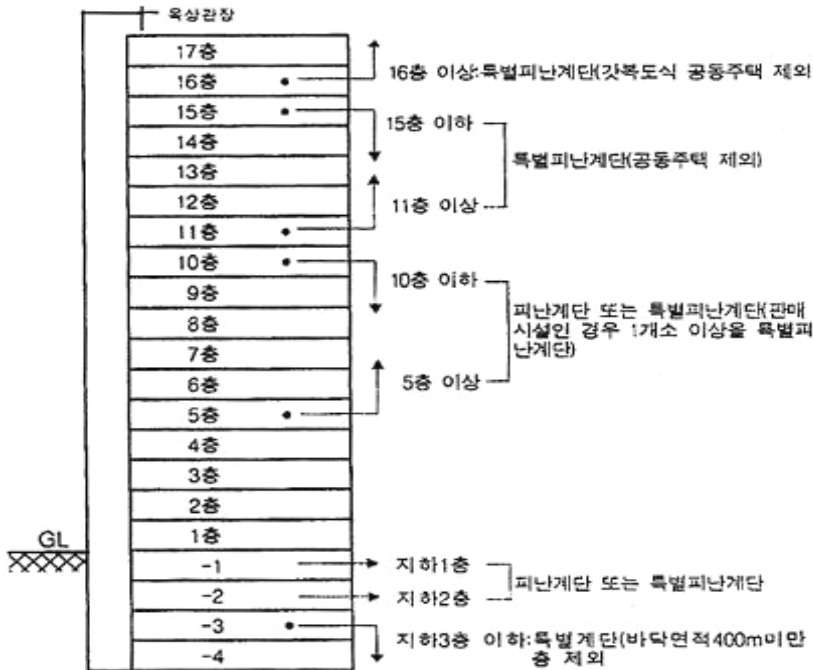
[그림 35] 피난계단 설치기준
