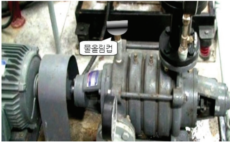
(그림 3-31) 후트밸브 고장여부 점검
