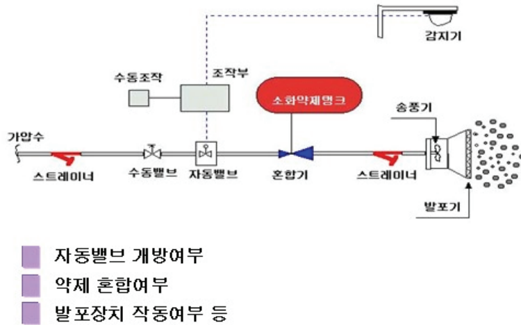
(그림 5-27) 고발포형 고정포 방출구 점검
