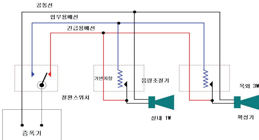
(그림 4) 3선식 배선의 결선
