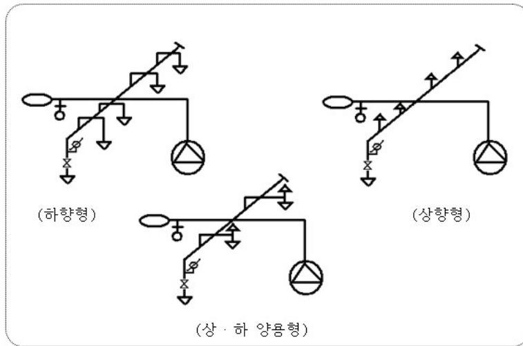
[그림 4-16] 헤드설치방법
