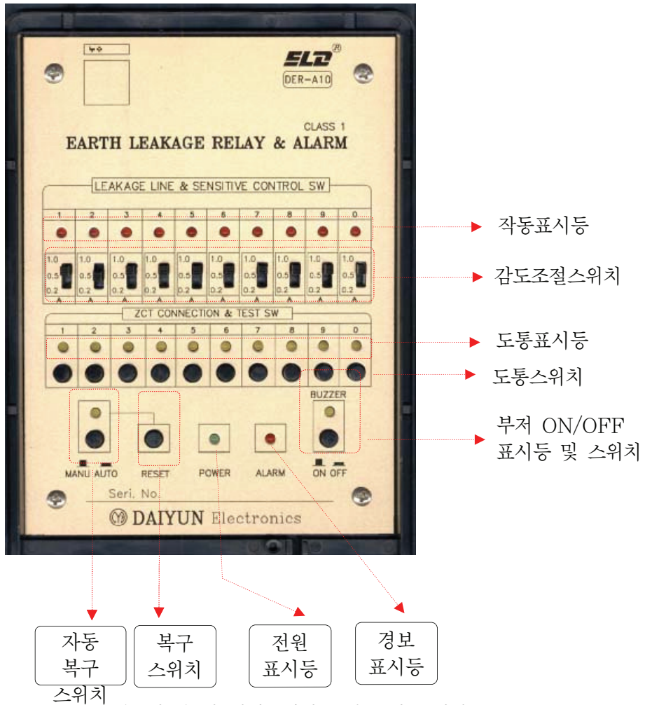
(그림 4) 누전경보기의 표시등 및 스위치
