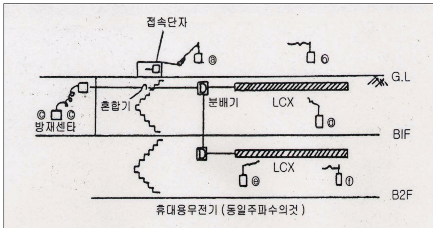
[그림 4] 무선통신보조설비의 사용
