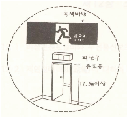
[그림 3] 피난구유도등 설치위치
