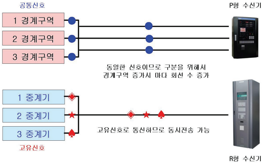
(그림 3) 공통신호와 고유신호의 구분
