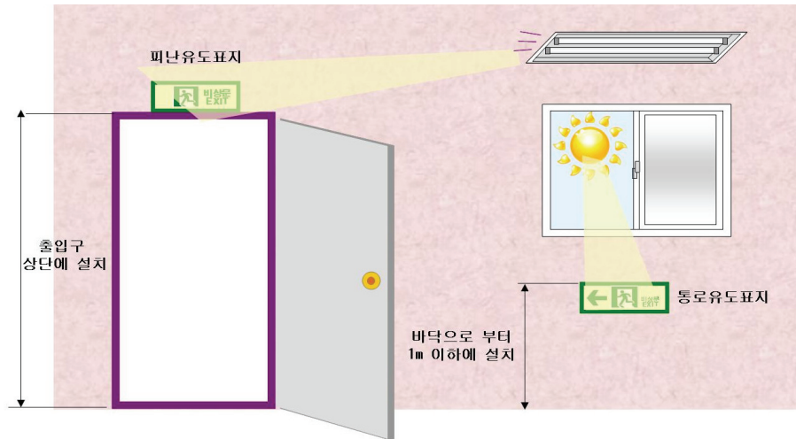
(그림 7) 유도표지 설치기준
