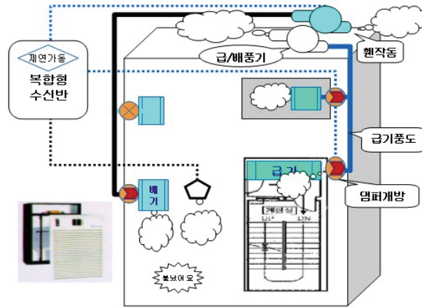
(그림 7-7) 부속실 제연설비 작동
