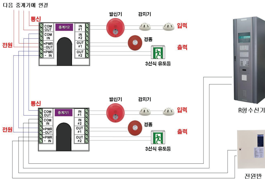
(그림 57) 분산형 중계기 계통배선
