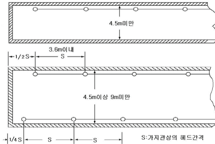
[그림 4-22] 측벽형 헤드설치
