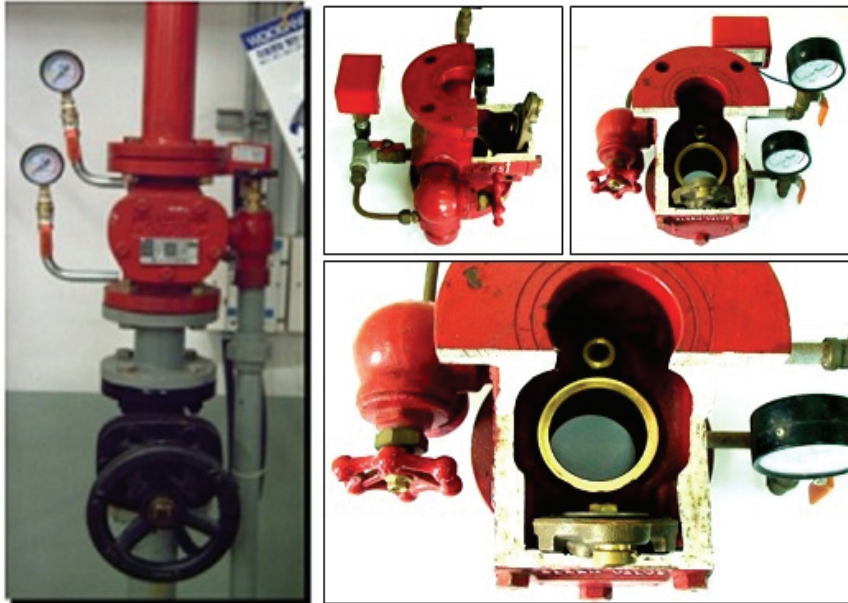
[그림 4-3] 습식밸브 구조
