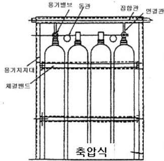
(그림 6-8) 축압식 저장방식
