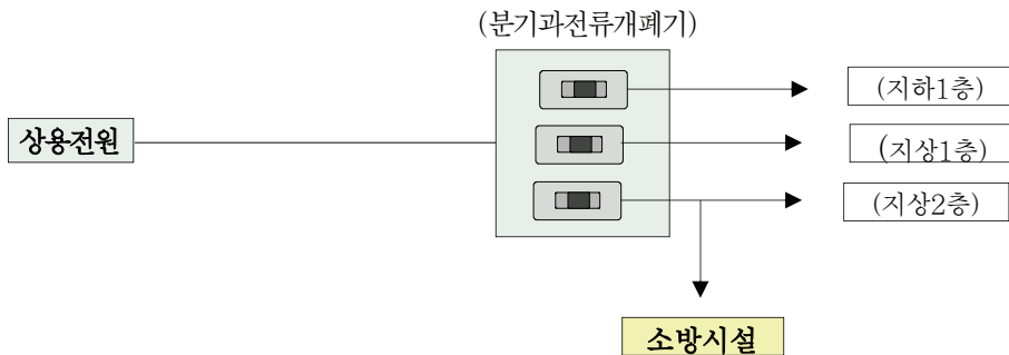
[그림 2] 소방시설 상용전원의 분기(×)
