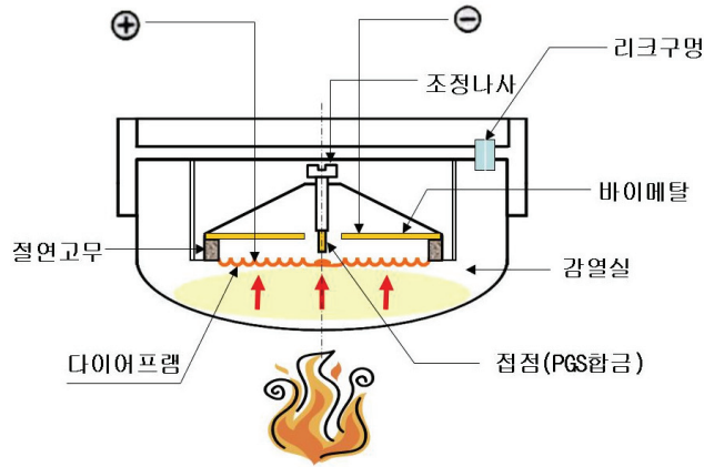
[그림 18] 보상식감지기 구조
