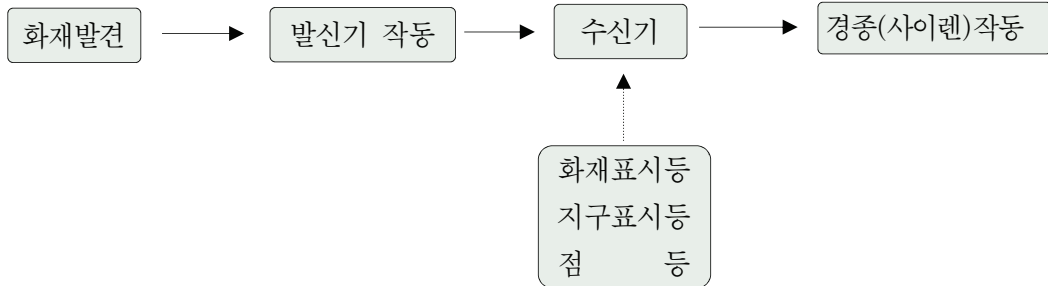
[그림 2] 비상벨설비의 작동흐름도
