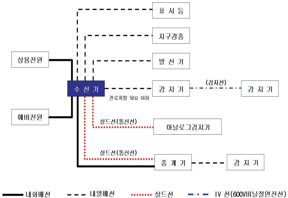
(그림 7) 자동화재탐지설비 구간배선
