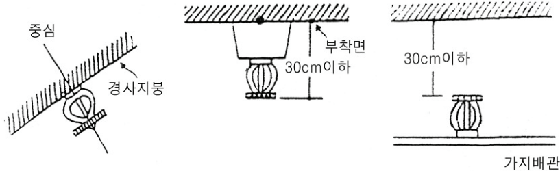
[그림 4-19] 헤드설치 살수방법
