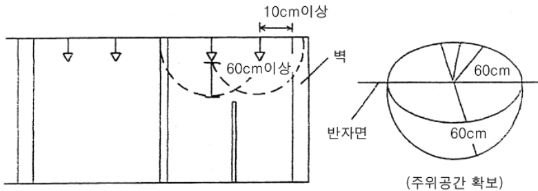
[그림 4-18] 헤드설치 살수반경
