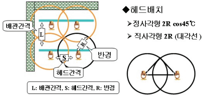
[그림 4-17] 정사각형 헤드배치 방법
