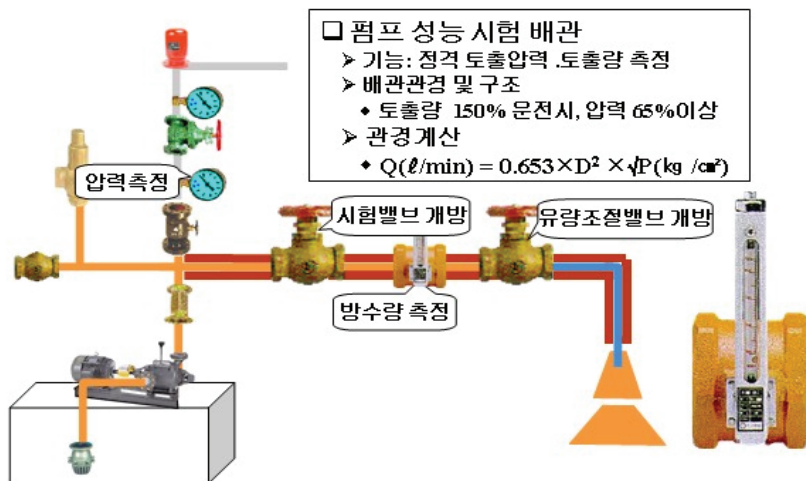
(그림 3-15) 펌프성능시험 배관
