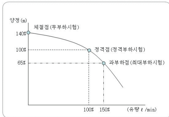
[소방펌프의 특성곡선]
