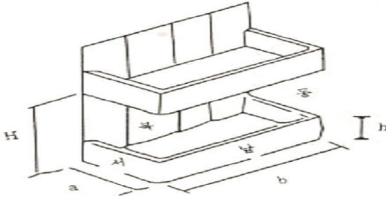
[그림 9] 노대등의 바닥면적 산정방법(1)
