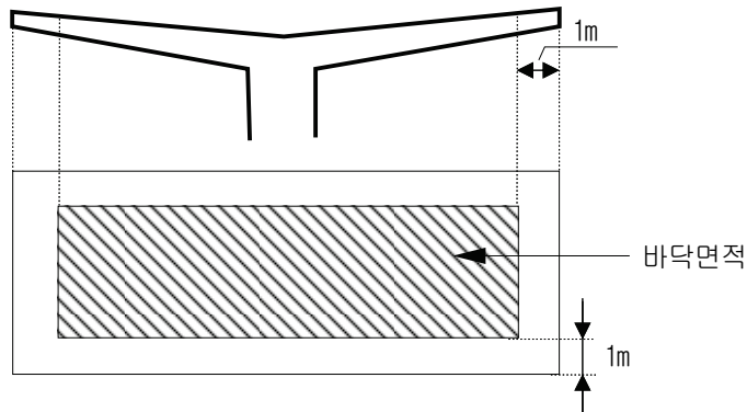
(그림 8) 벽·기둥의 구획이 없는 건축물의 바닥면적 산정방법
