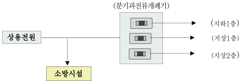
(그림 3) 소방시설 상용전원의 분기(○)
