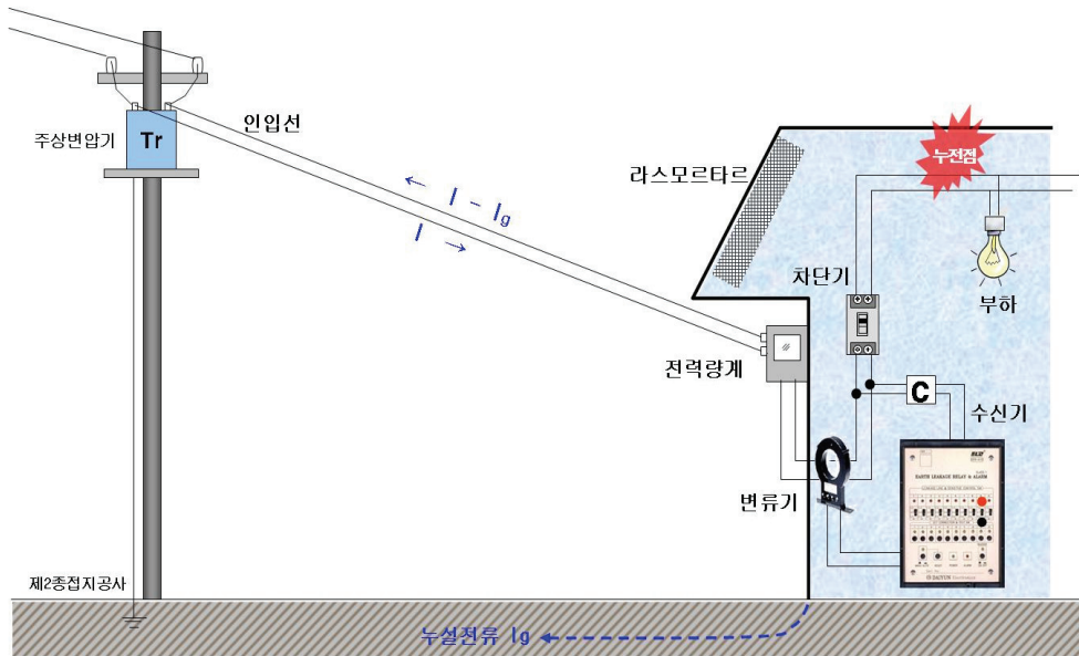
[그림 2] 누전경보기 설치구성도
