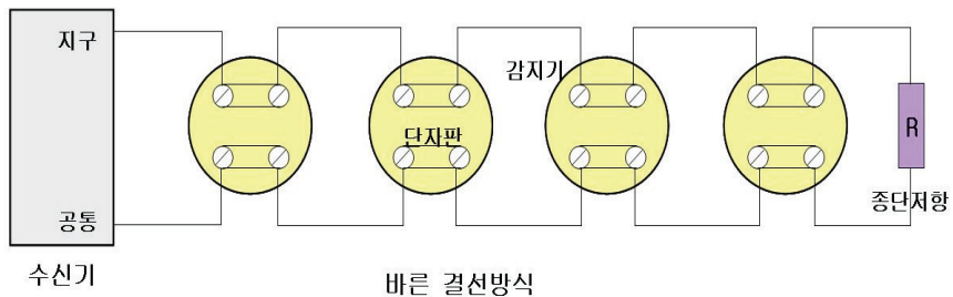
(그림 54) 감지기 배선 송배선방식
