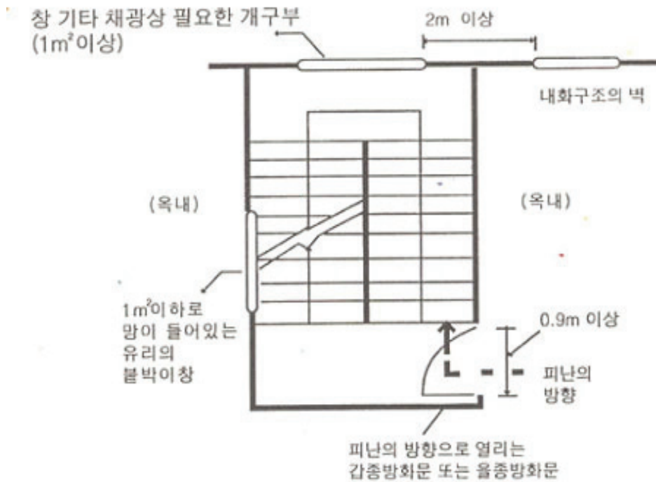
[그림 36] 옥내피난계단의 구조
