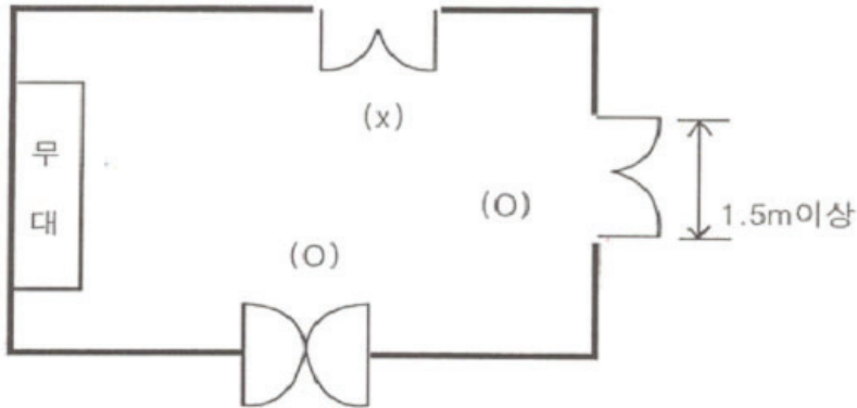
(그림 29) 출구의 문 설치기준
