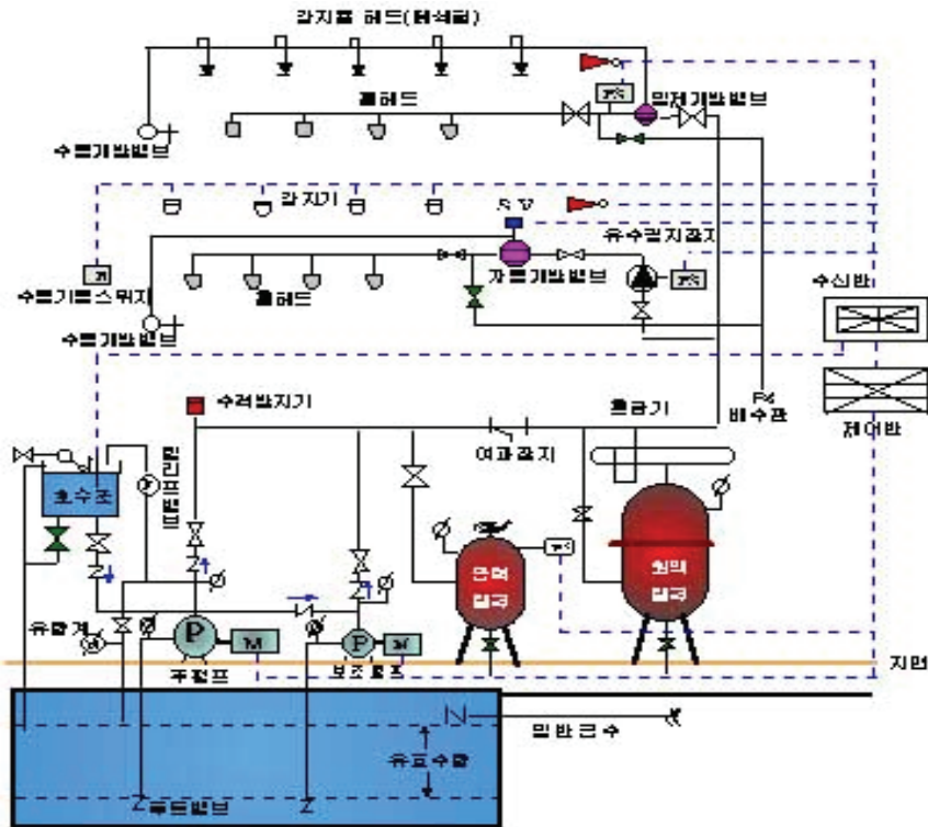
(그림 5-13) 홈헤드설비 방식
