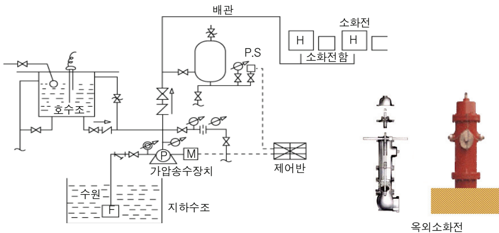
[그림 3-29] 옥외소화전 계통도
