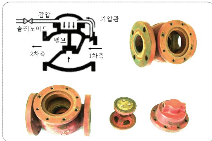
[그림 4-13] 일제개방밸브 구조
