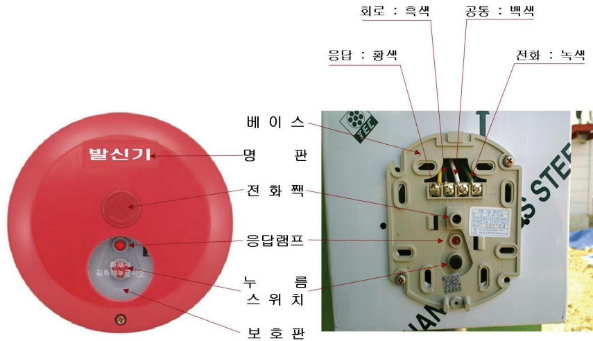
(그림 38) 발신기 구성
