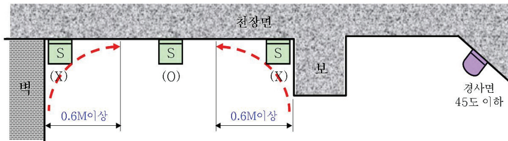
(그림 32) 벽 및 보로부터의 감지기의 설치위치
