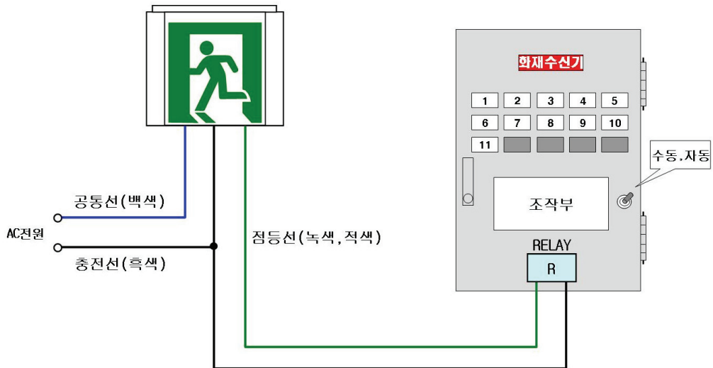
[그림 11] 3선식 유도등의 배선
