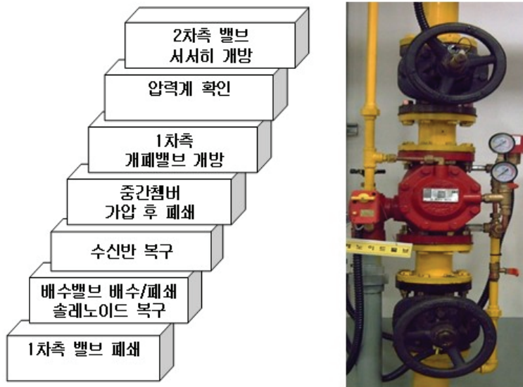
(그림 4-28) 준비작동식 복구순서
