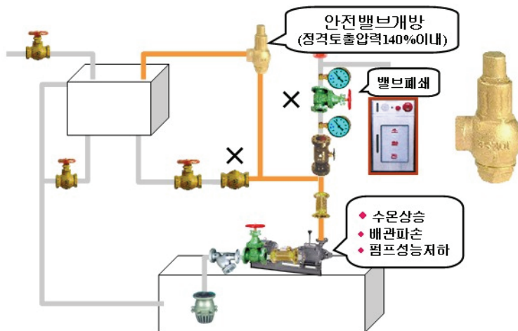
(그림 3-11) 순환배관 구조와 기능
