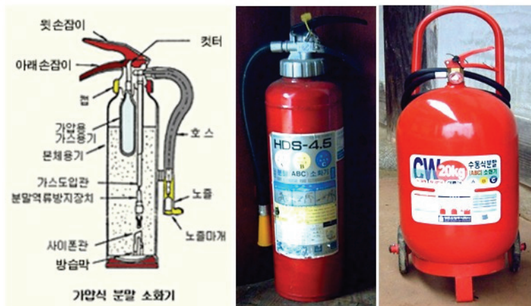
(그림 2-3) 가압식 분말소화기 구조
