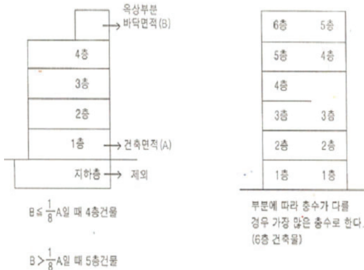
(그림 19) 건축물의 층수산정
