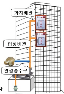
(그림 3-17) 배관 및 송수구
