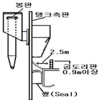
(그림 5-16) 특형 방출구
