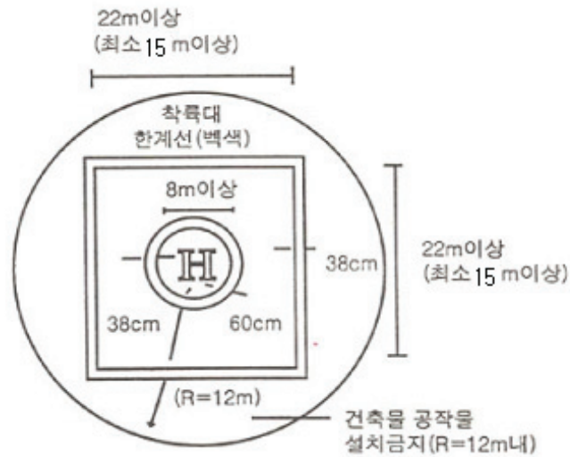
[그림 39] 헬리포트의 설치기준
