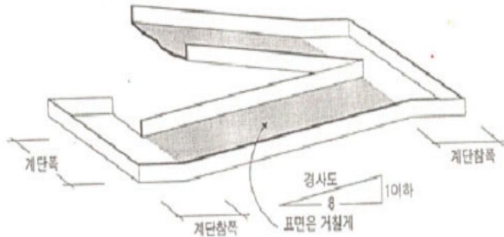
[그림 31] 경사로의 기준
