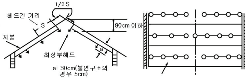
(그림 4-20) 경사지붕의 헤드설치
