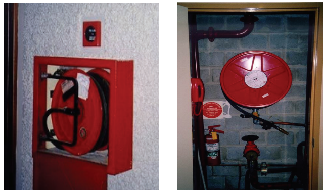
(그림 3-28) 호스릴옥내소화전 설비
