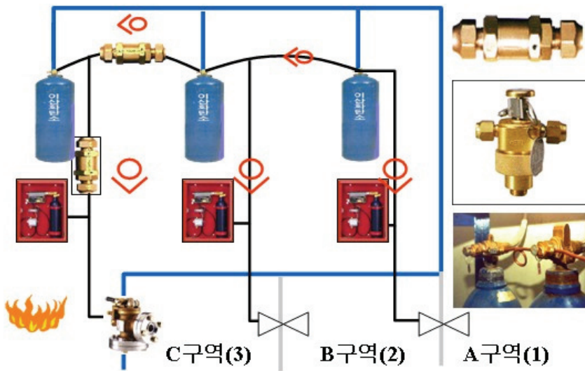
(그림 6-3) 방호구역과 선택밸브
