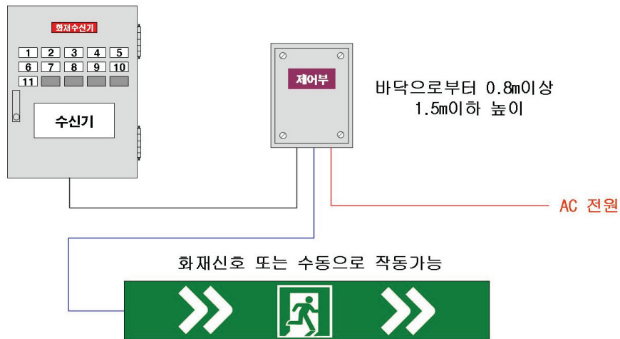
(그림 8) 광원점등방식 피난유도선 구성도
