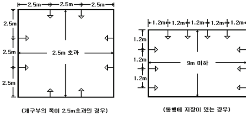
(그림 4-21) 연소할 개구부의 헤드설치
