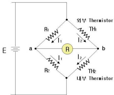
휘트스톤 브리지 회로
