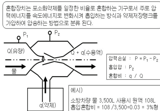
(그림 5-5) 포소화약제 혼합장치
