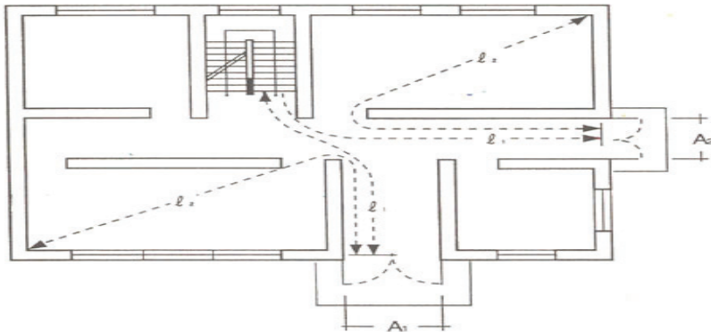
(그림 30) 거실 및 직통계단에서 옥외로의 출구까지 보행거리 기준
