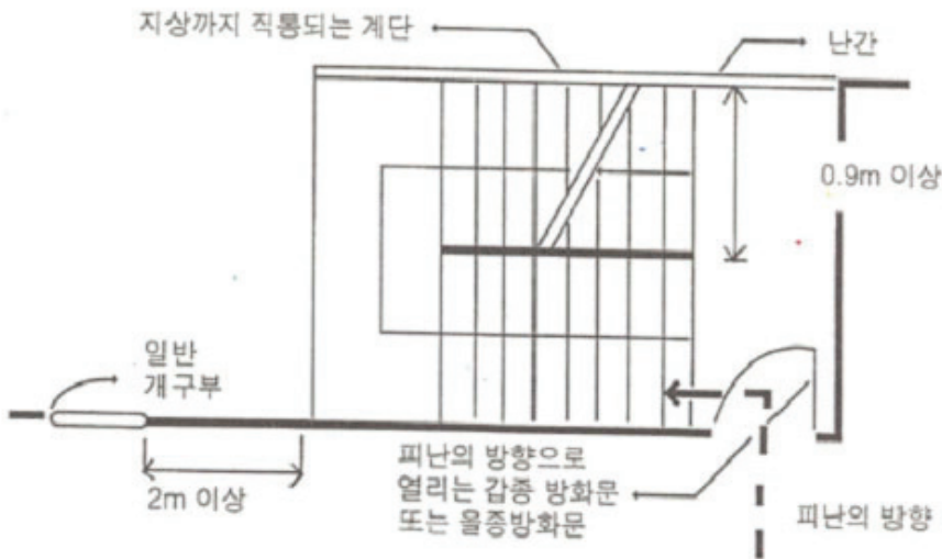
(그림 37) 옥외피난계단의 구조
