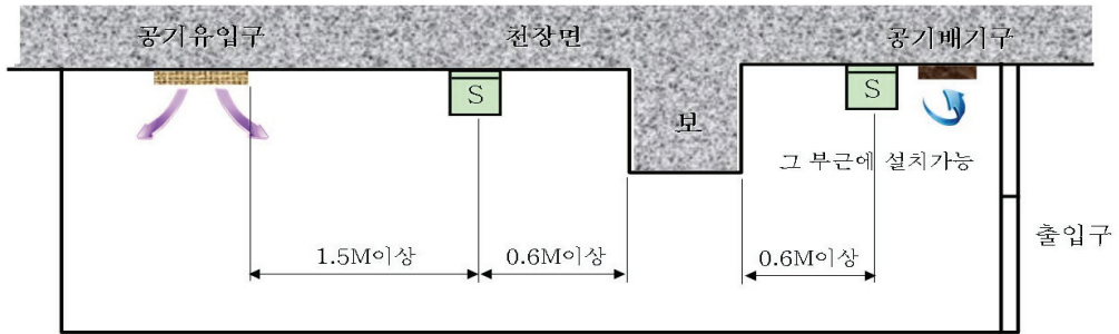
[그림 33] 연기감지기의 설치위치
