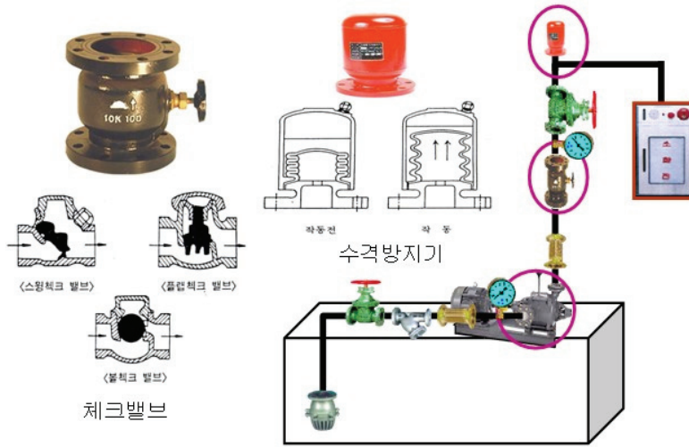
[그림 3-8] 체크밸브와 수격방지장치
