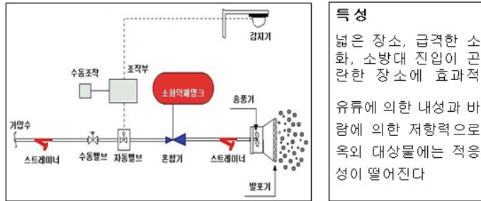
(그림 5-19) 고발포형 고정포 방출구
