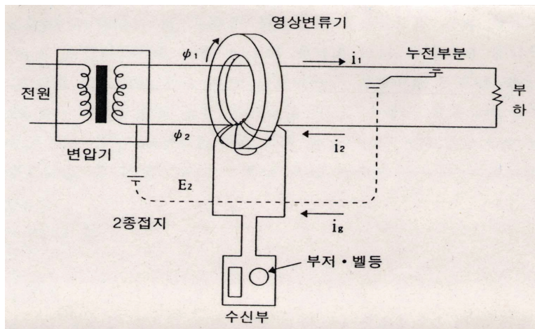
(그림 3) 누전경보기의 작동원리
