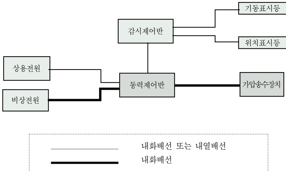
[그림 8] 소화전 구간배선
