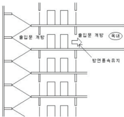
(그림 7-11) 방연풍속 측정
