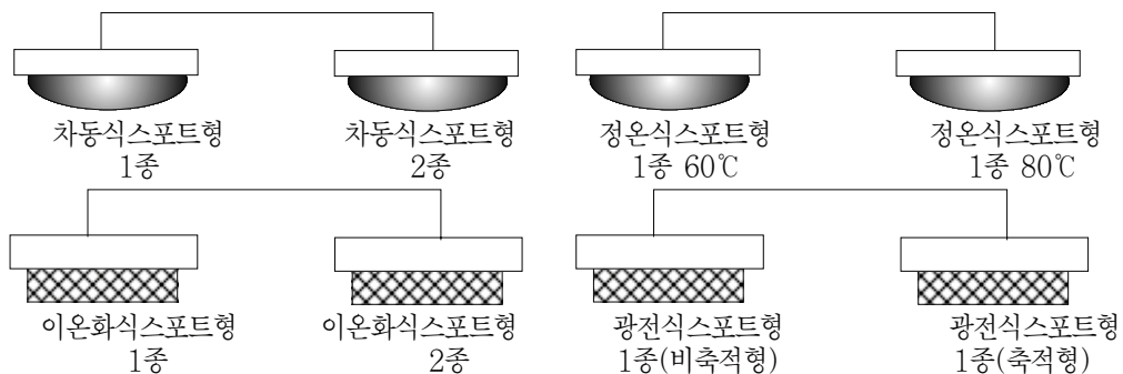
[그림 29] 다신호식감지기의 구성
