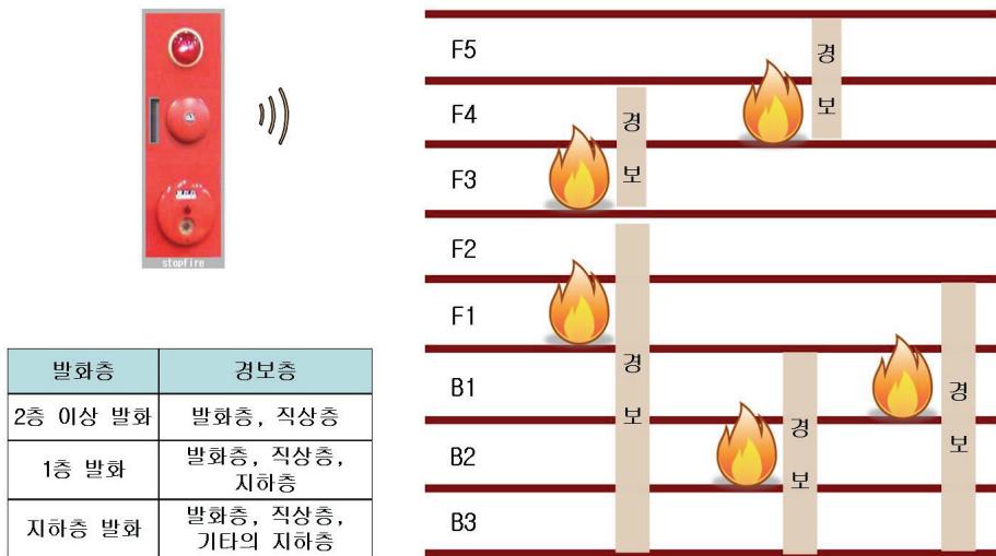
(그림 44) 직상발화우선경보방식 경보장치 작동
