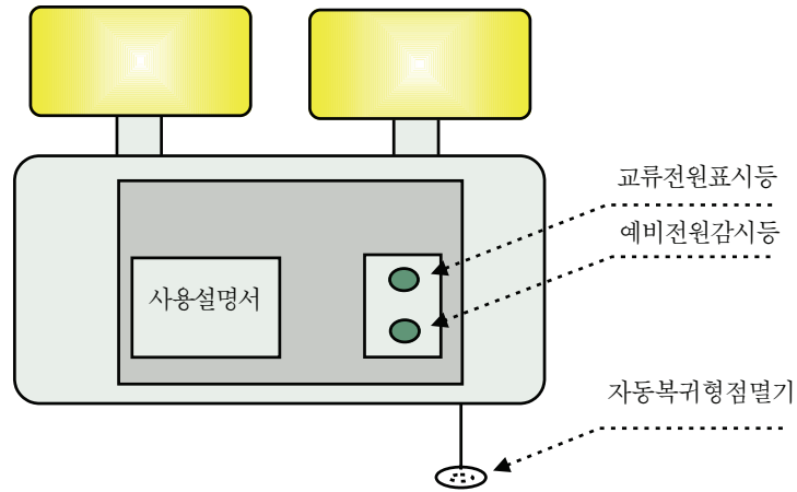
(그림 3) 비상조명등 표시등 및 스위치
