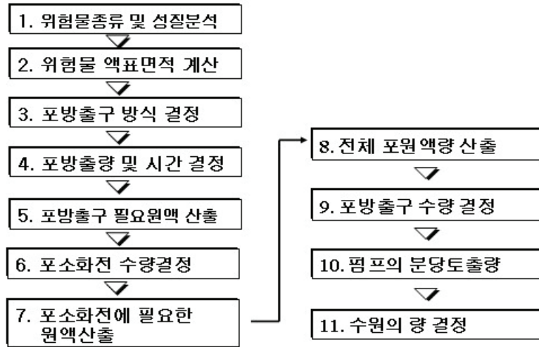
(그림 5-25) 옥외탱크 포소화전설비 설계 검토
