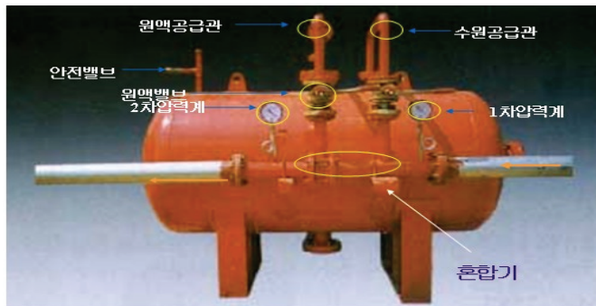
[그림 5-10] 포원액 탱크
