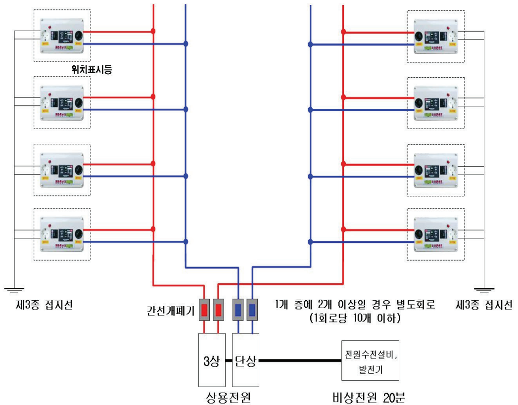
[그림 2] 비상콘센트설비의 배선도
