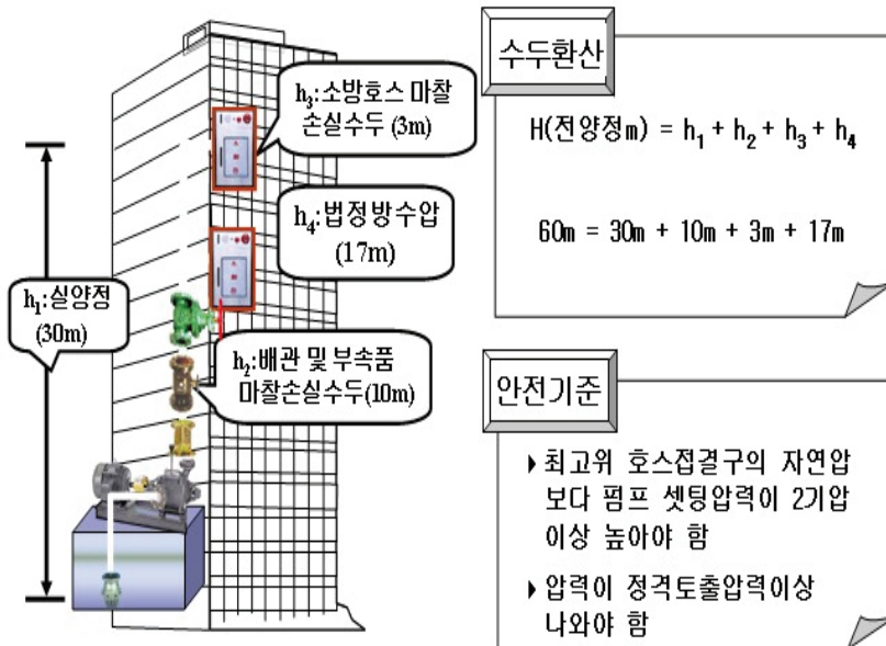
(그림 3-19) 양정계산과 압력셋팅
