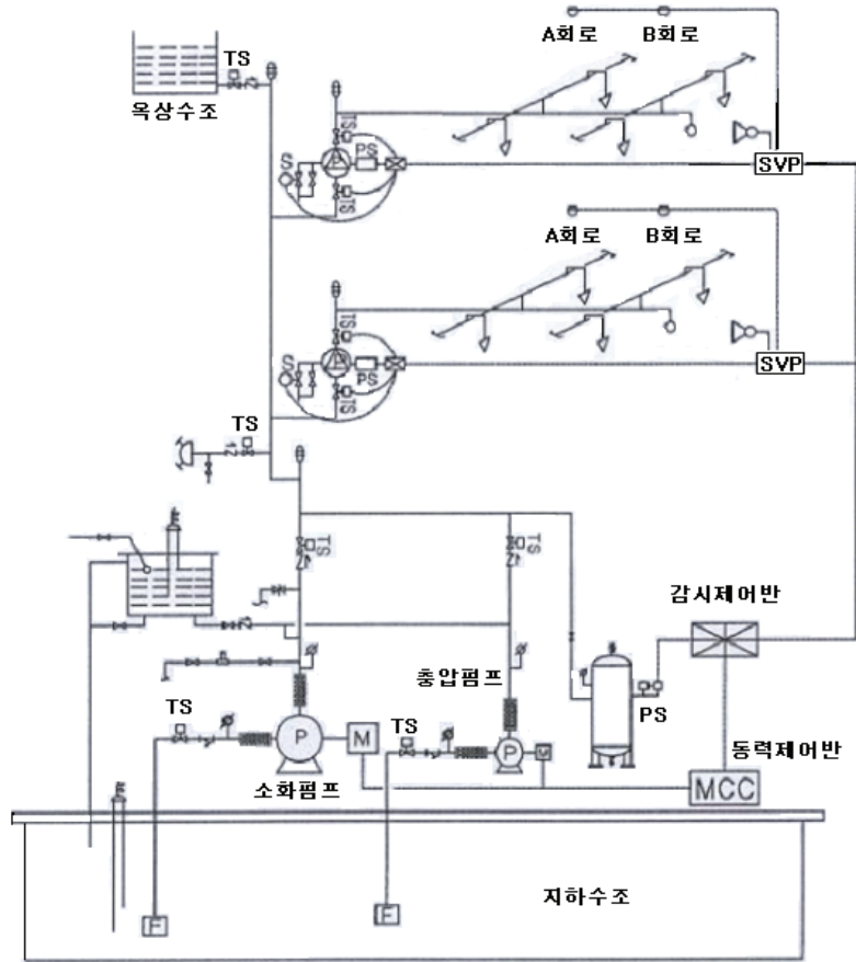
(그림 4-1) 준비작동식 스프링클러설비 계통도
