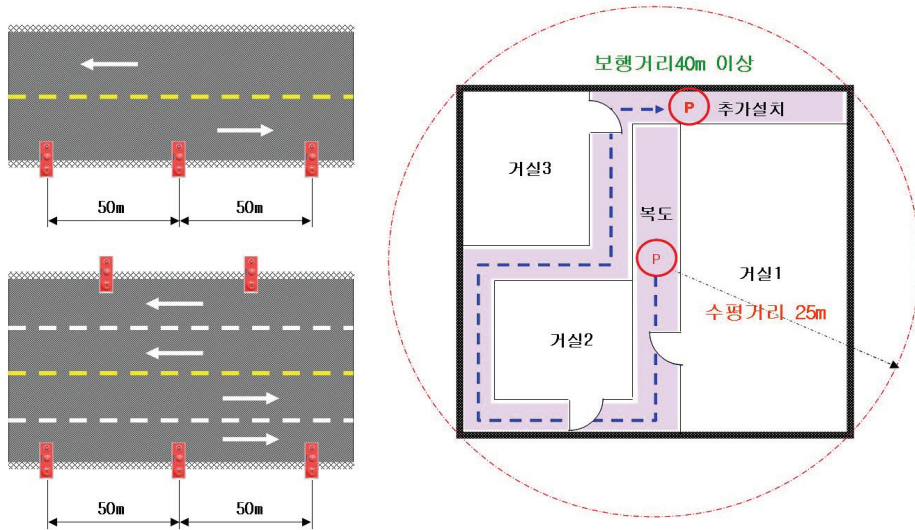
(그림 41) 터널 설치기준과 보행거리 초과시 추가설치
