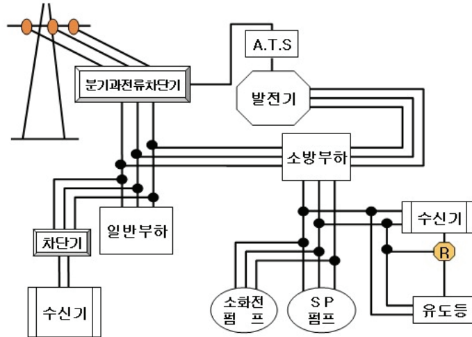
(그림3-23) 소방시설 전원 결선도
