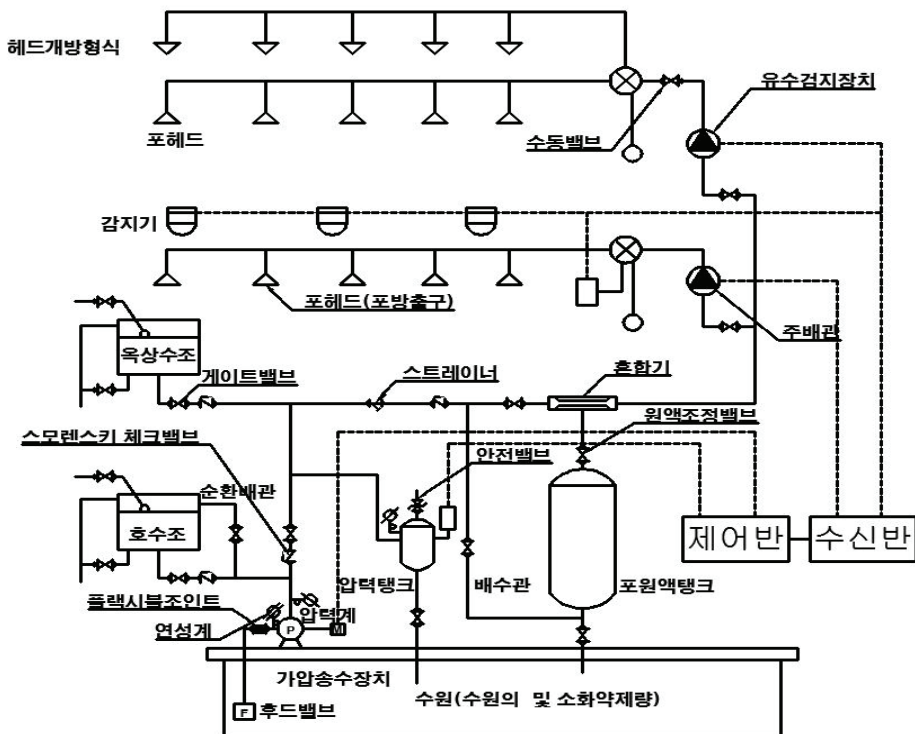
(그림 5-1) 포소화설비 계통도
