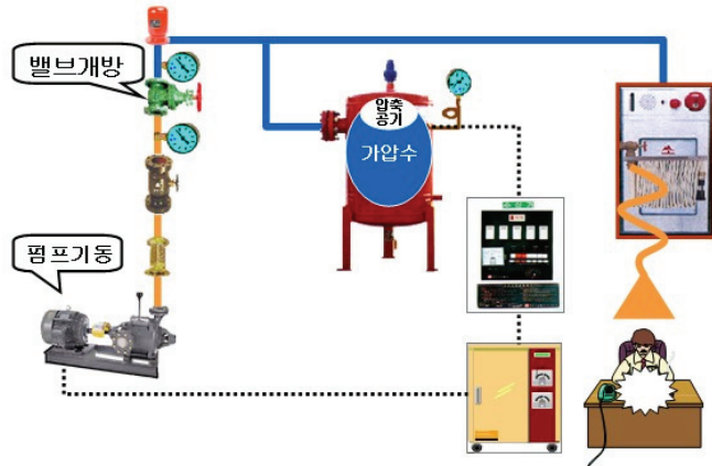
(그림 3-14) 압력챔버 구성과 기능
