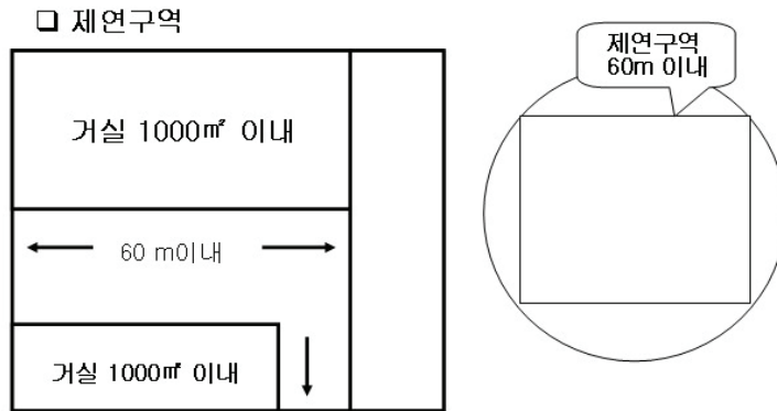
[그림 7-5] 제연구역 설정
