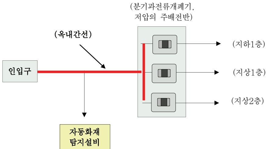
(그림 4) 자동화재탐지설비 상용전원의 분기
