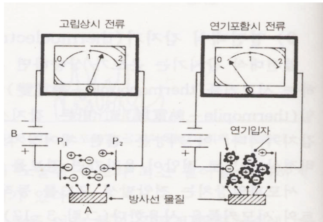
(그림 20) 이온화식감지기의 회로구성
