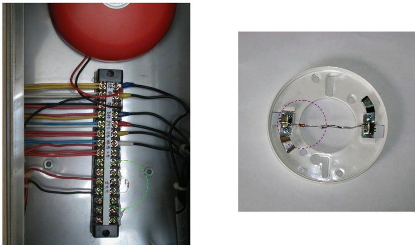
(그림 53) 중단저항 설치(발신기세트함 및 중단감지기)
