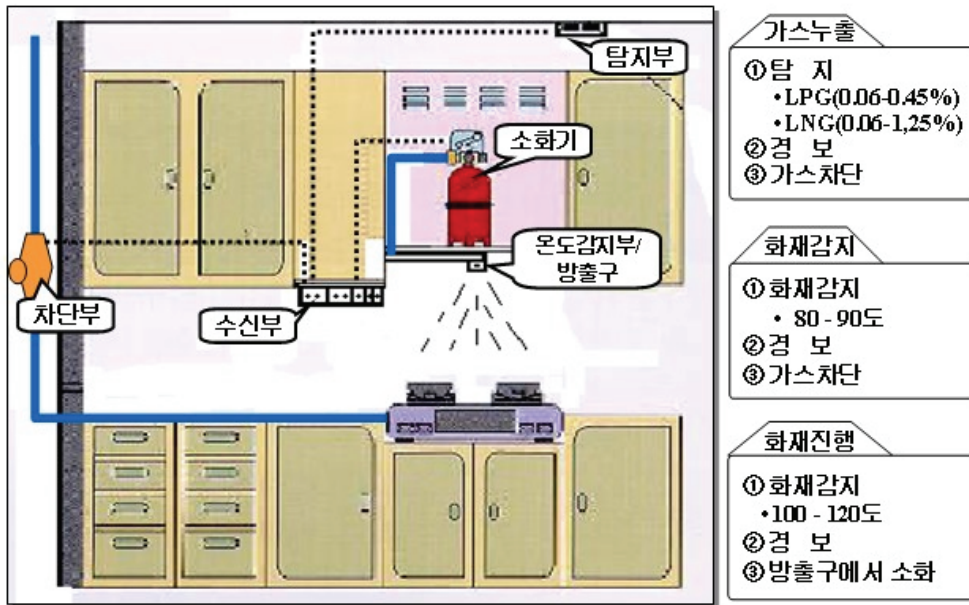
[그림 2-6] 자동식 소화기
