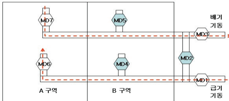
(그림 7-4) 화재시 제연설비로 전환
