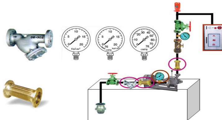
(그림 3-7) 흡입측 배관 부속품 및 밸브류
