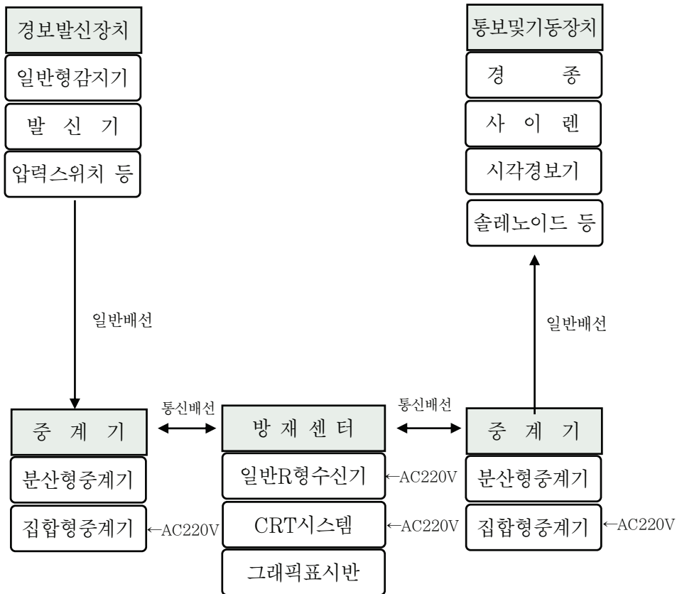
(그림 58) 중계기를 사용한 R형 시스템
