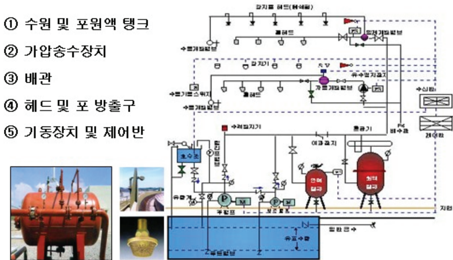
(그림 5-2) 포소화설비 구성요소
