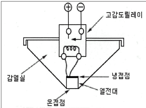
[그림11] 열전대식 감지기
