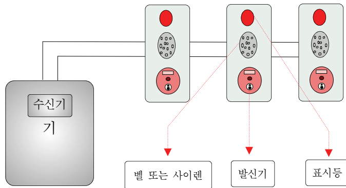
(그림 1) 비상벨/자동식사이렌설비의 구조
