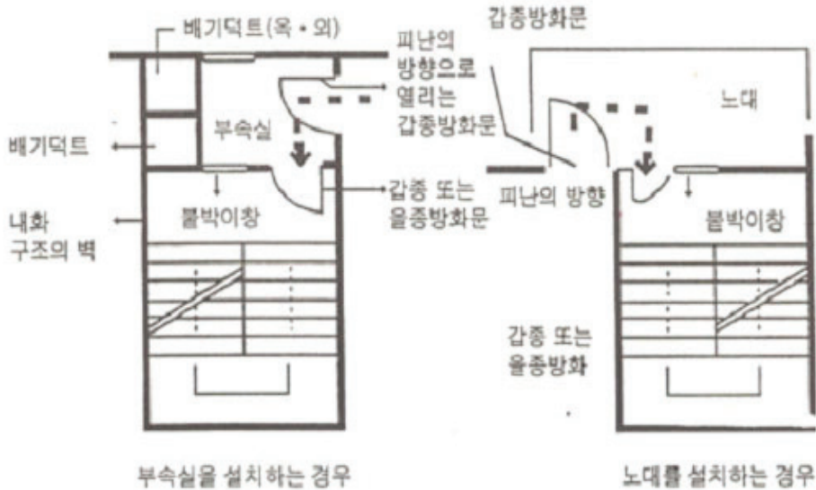
[그림 38] 특별피난계단의 구조
