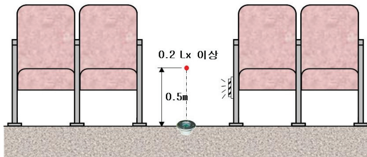
[그림 6] 객석유도등의 설치기준
