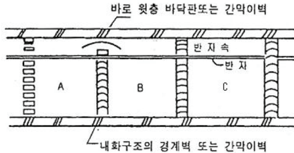
(그림 22) 경계벽 및 간막이벽의 설치방법
