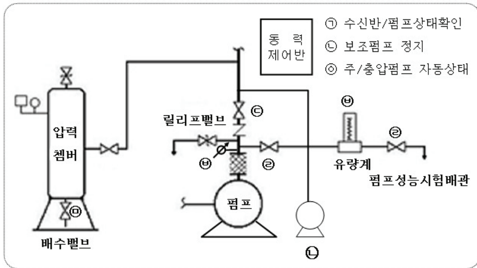
[그림 3-16] 펌프성능시험 방법
