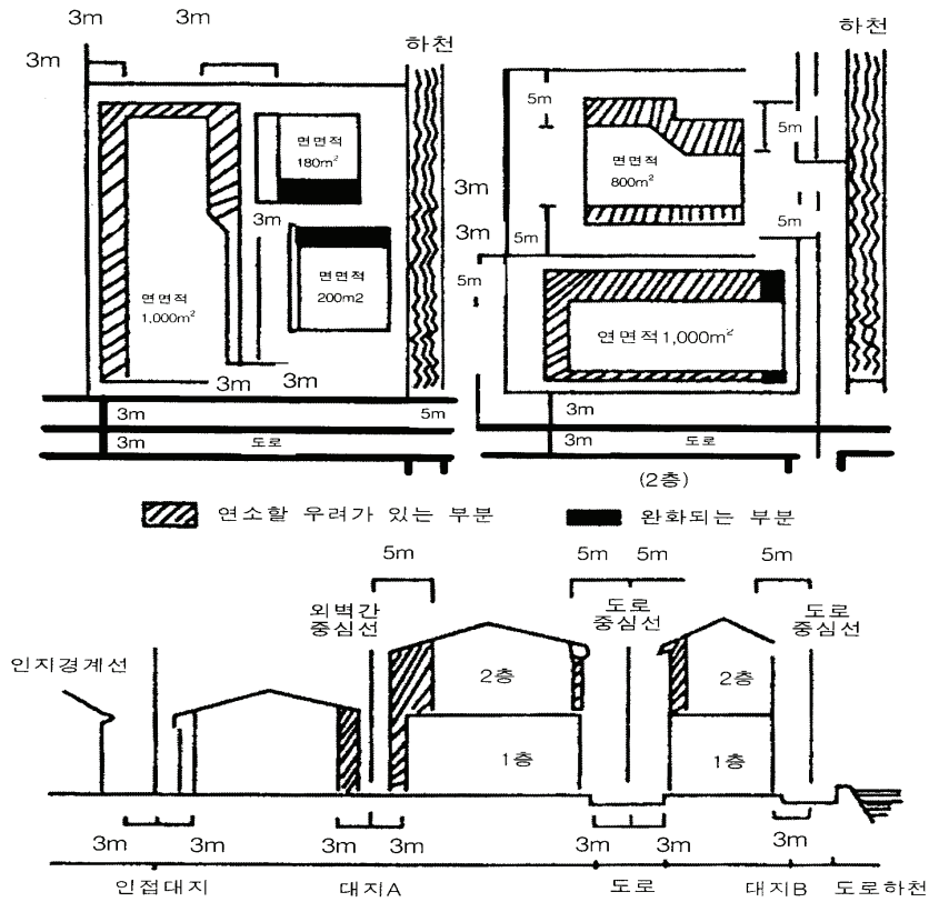
(그림 2) 연소할 우려가 있는 부분
