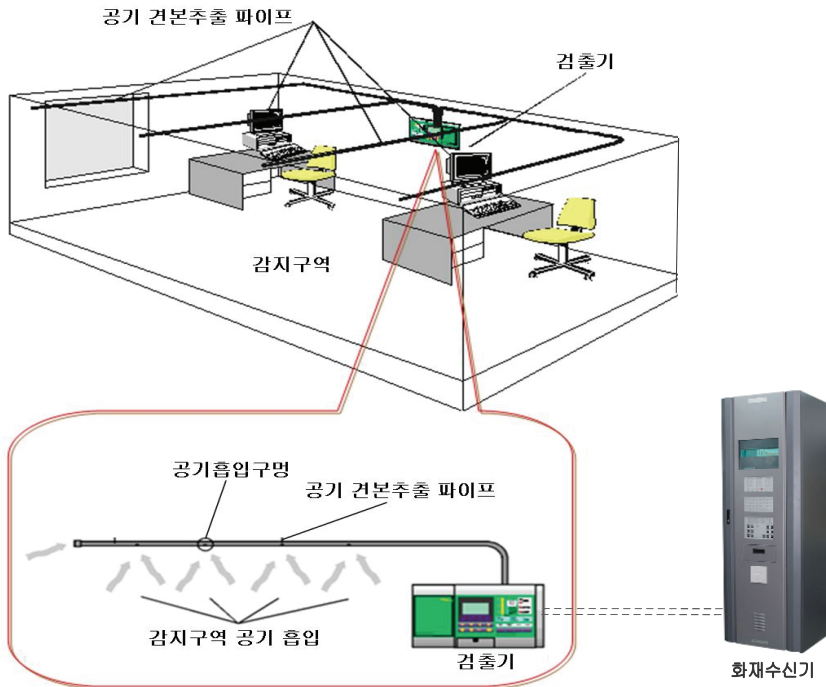
(그림 25) 광전식 공기흡입형감지기의 구성
