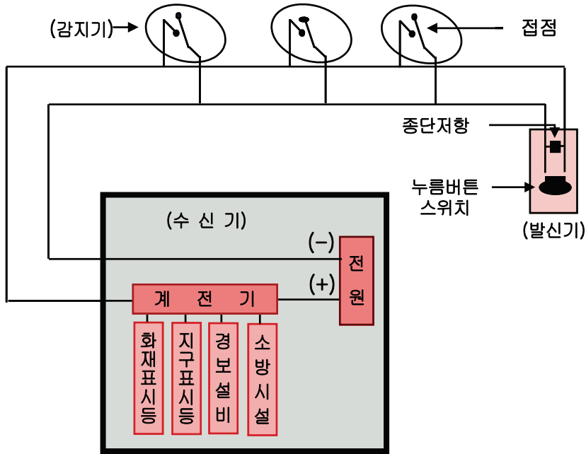
(그림 2) 자동화재탐지설비의 회로 간략도
