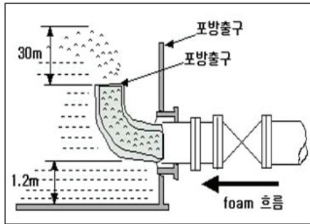
(그림 5-17) 표면하 주입구
