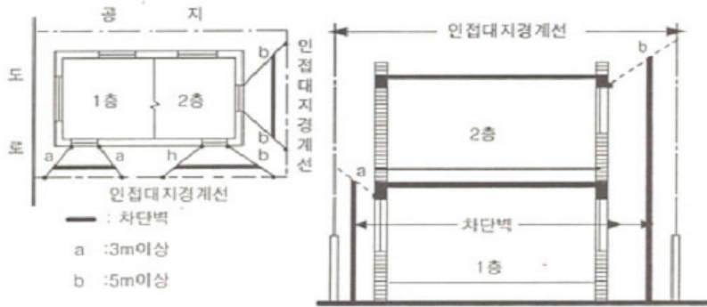
(그림 23) 차단벽 설치
