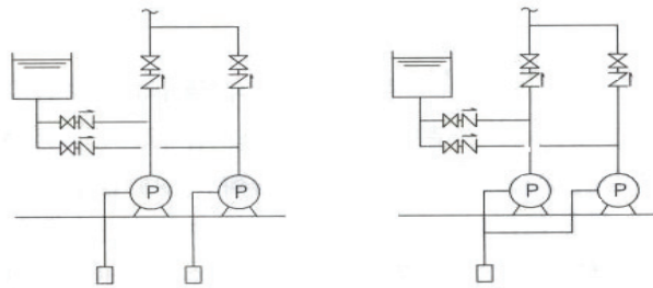
[올바른 시공]
