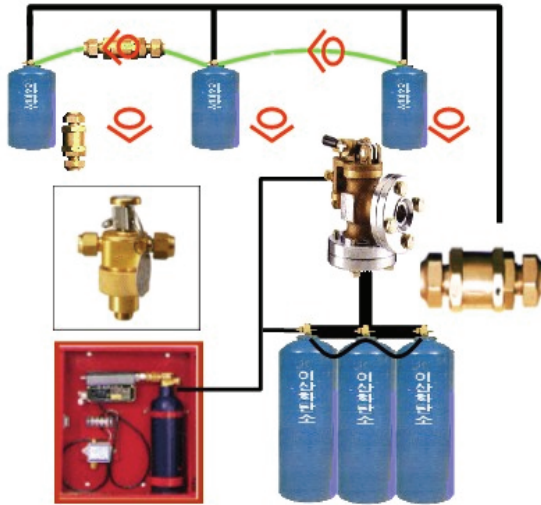
(그림 6-11) 저장용기 점검
