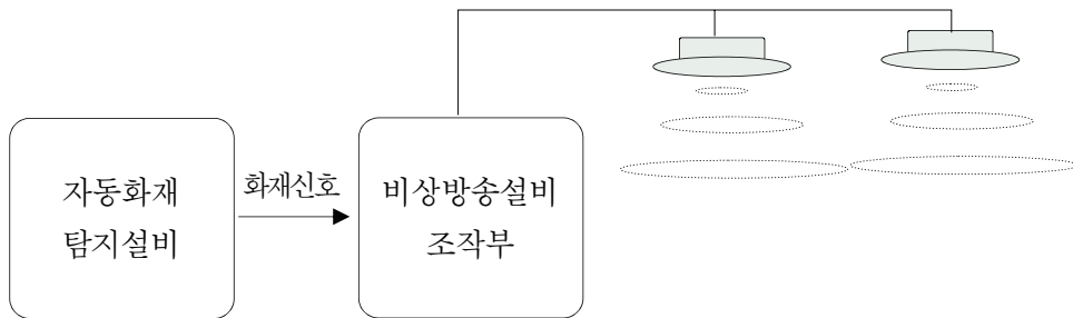
(그림 2) 비상방송설비의 작동흐름도
