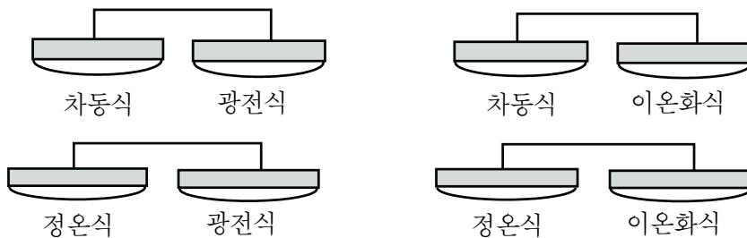
(그림 28) 열연복합형감지기의 구성
