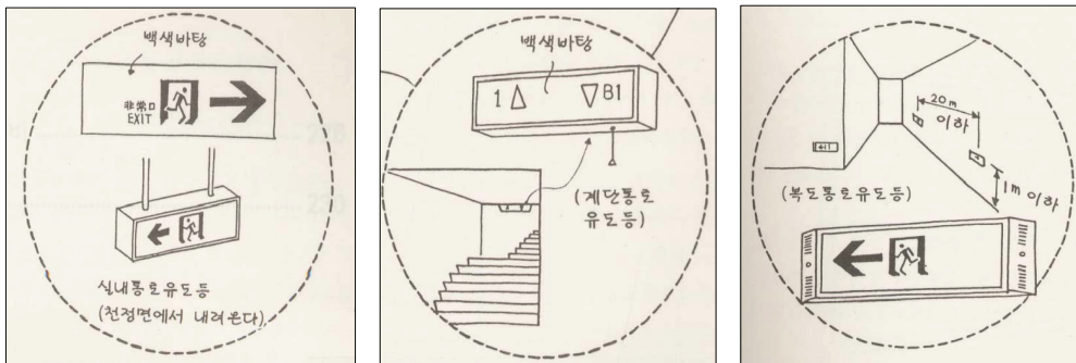
(그림 5) 통로유도등의 설치 기준
