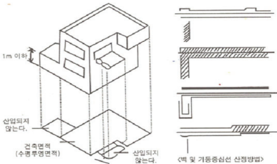
[그림 7] 건축면적의 산정방법
