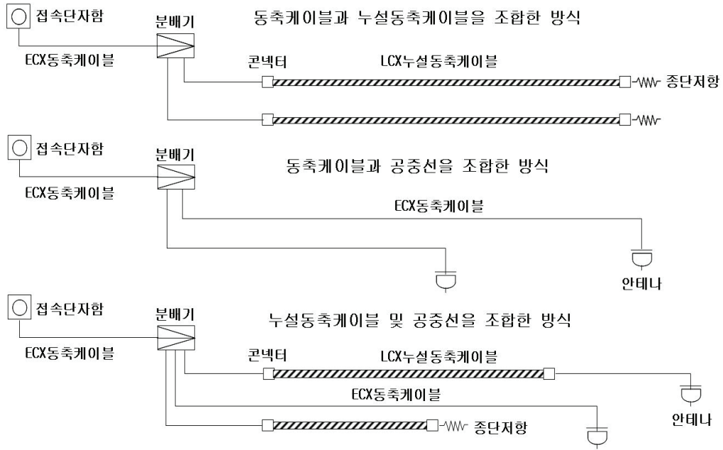
(그림 5) 무선통신보조설비의 종류
