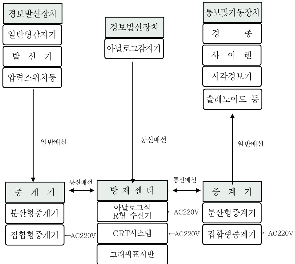
(그림 59) 아날로그식 감지기를 사용하는 경우
