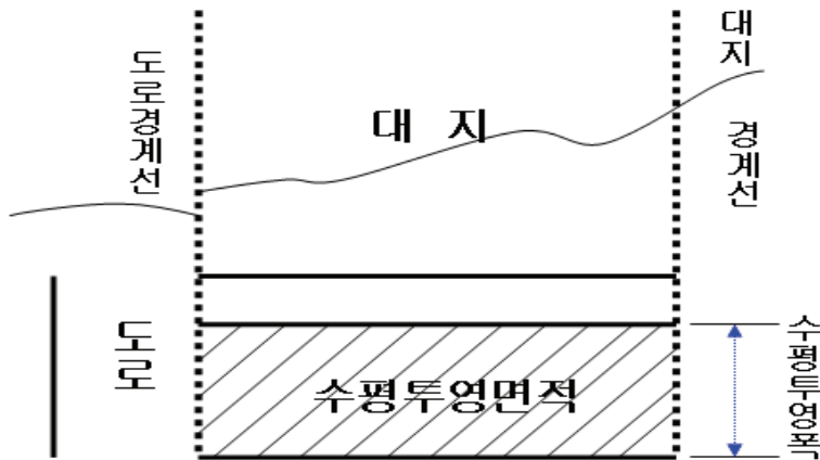
(그림 4) 대지면적의 산정방법(1)
