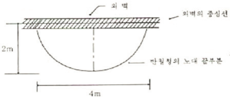
[그림 10] 노대등의 바닥면적 산정방법(2)
