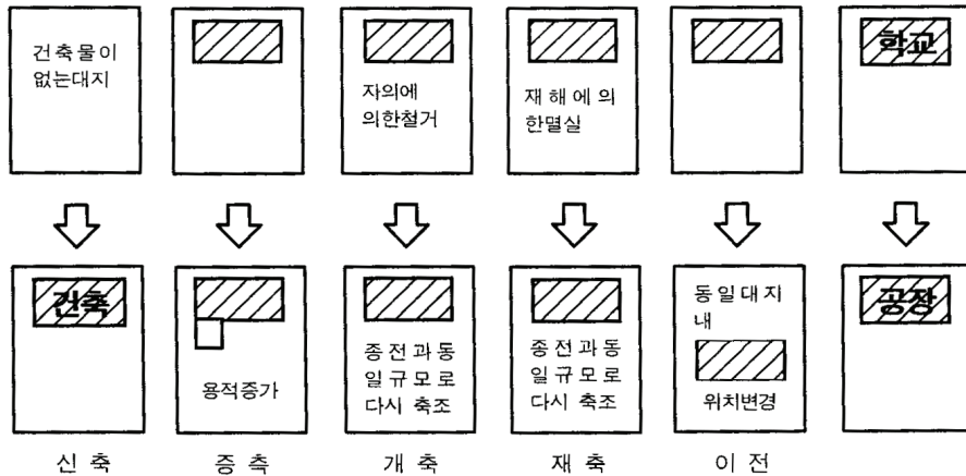
(그림 3) 건축 행위
