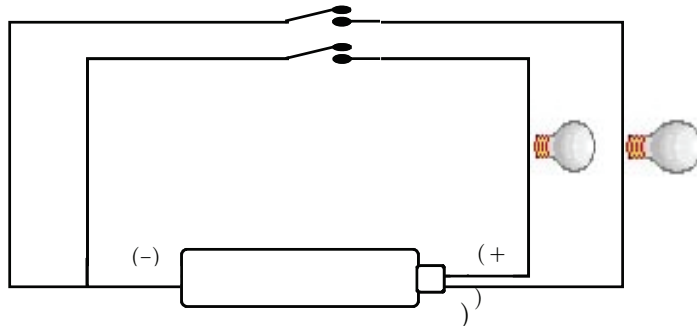
(그림 52) 공통선 배선
