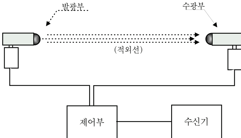
[그림 24] 광전식분리형감지기
