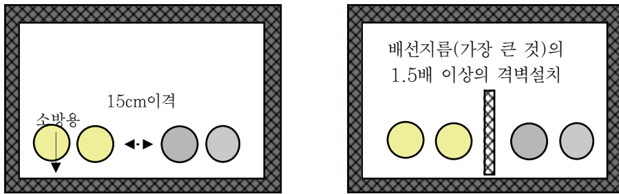
[그림 6] 내화배선 공사방법
