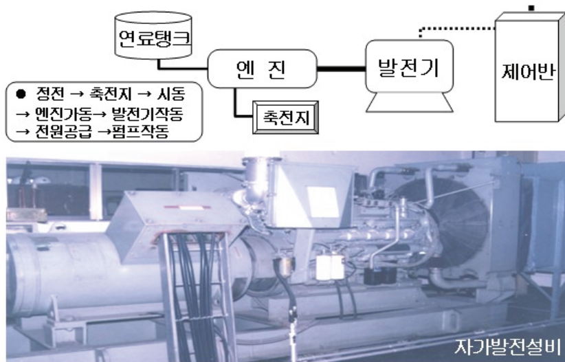
(그림 3-27) 자가발전설비
