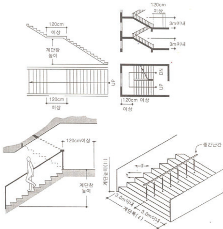
[그림 33] 계단의 설치기준
