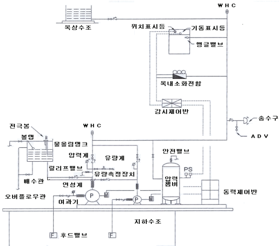
(그림 3-1) 옥내소화전 계통도 5)
