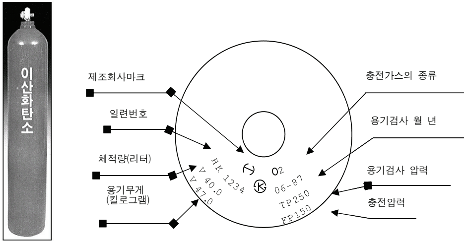
[그림 6-6] 가스저장용기
