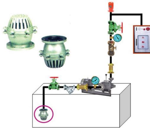
(그림 3-5) 가압송수장치 펌프방식
