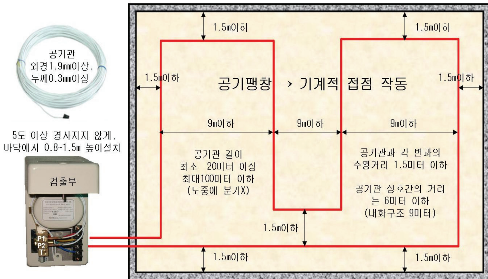
(그림 34) 공기관식 감지기의 설치기준
