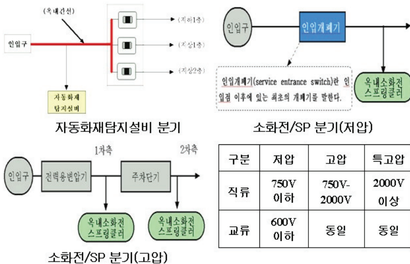
(그림 3-24) 상용전원 분기방식
