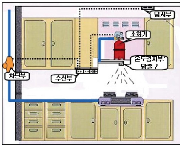
(그림 2-12) 자동식 소화기 점검
