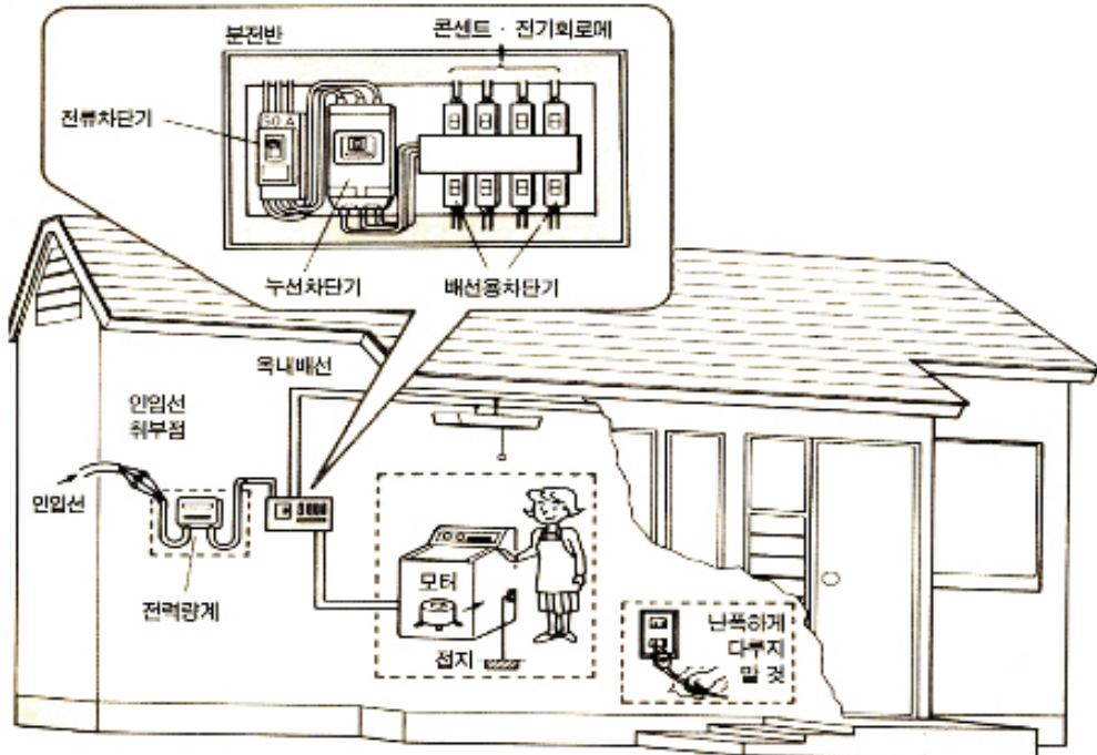
(그림 3-22) 상용전원 결선도
