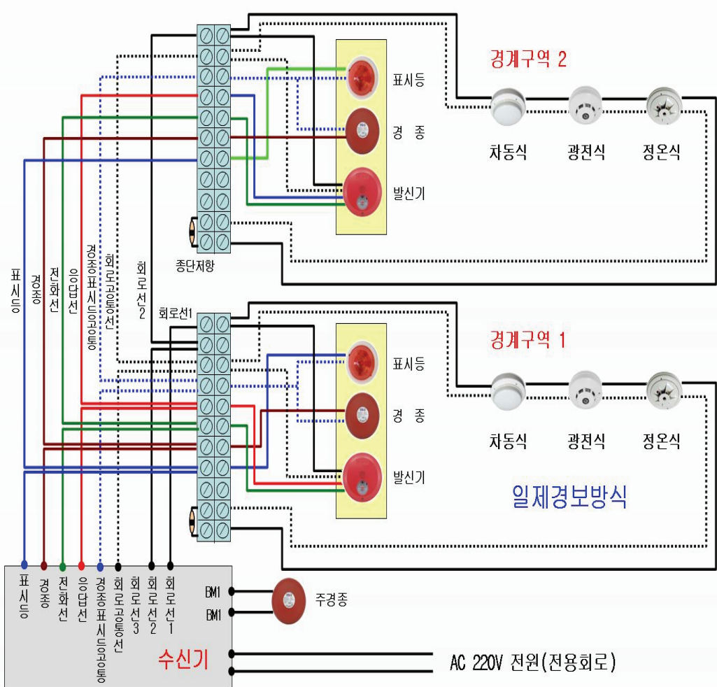
[그림 55] 여러 경계구역의 연결
