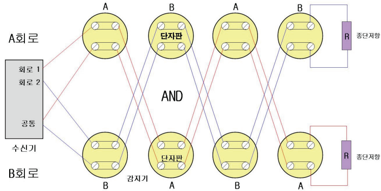
(그림 47) 자동소화설비 화재감지기용 회로는 교차회로
