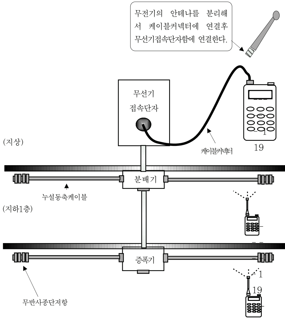
[그림 2] 무선통신보조설비의 구성
