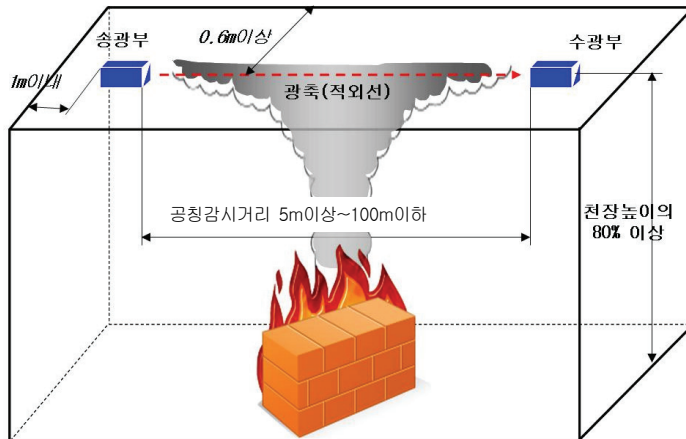
(그림 36) 광전식분리형감지기의 설치기준
