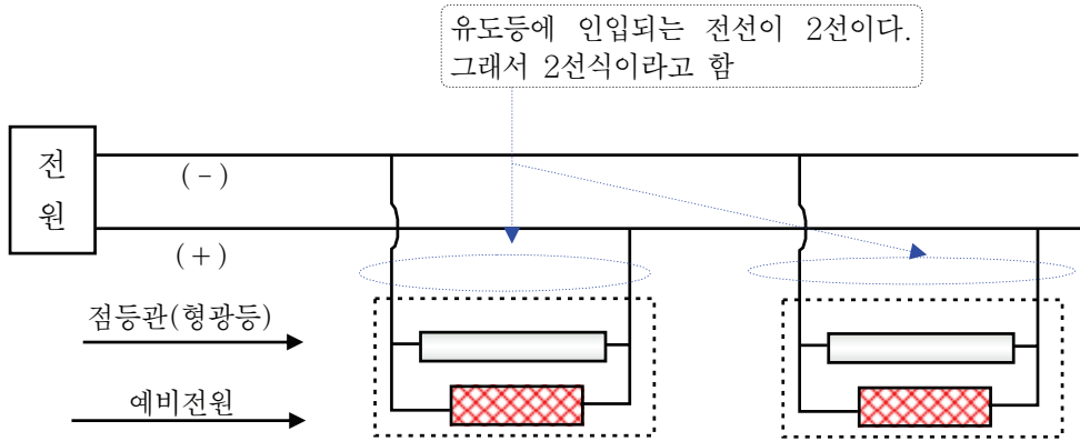
[그림 10] 2선식유도등의 배선
