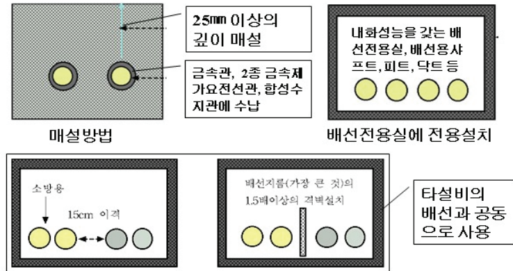
(그림 3-25) 내화배선 공사방법
