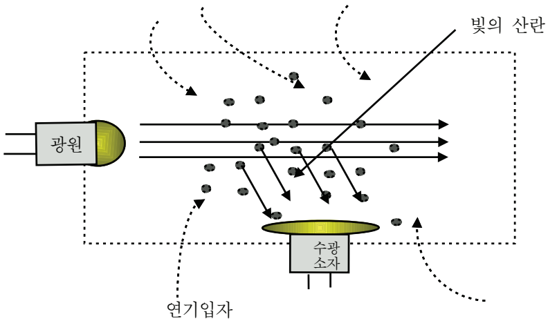
[그림 21] 감광식의 감지원리
