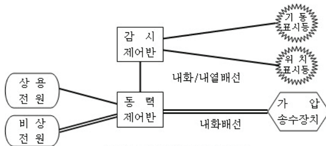
[옥내소화전/SP설비의 배선]
