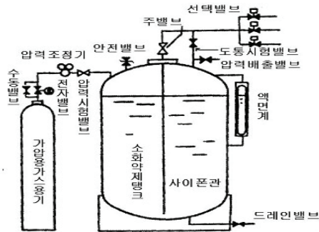
(그림 6-9) 가압식 저장방식
