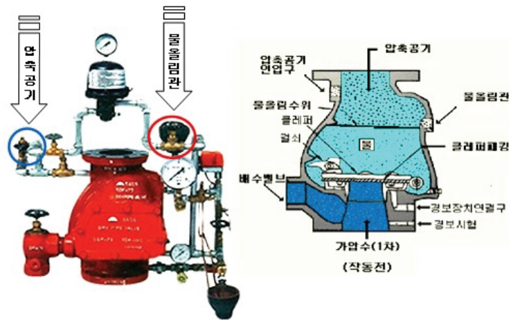
(그림 4-10) 건식밸브 구조
