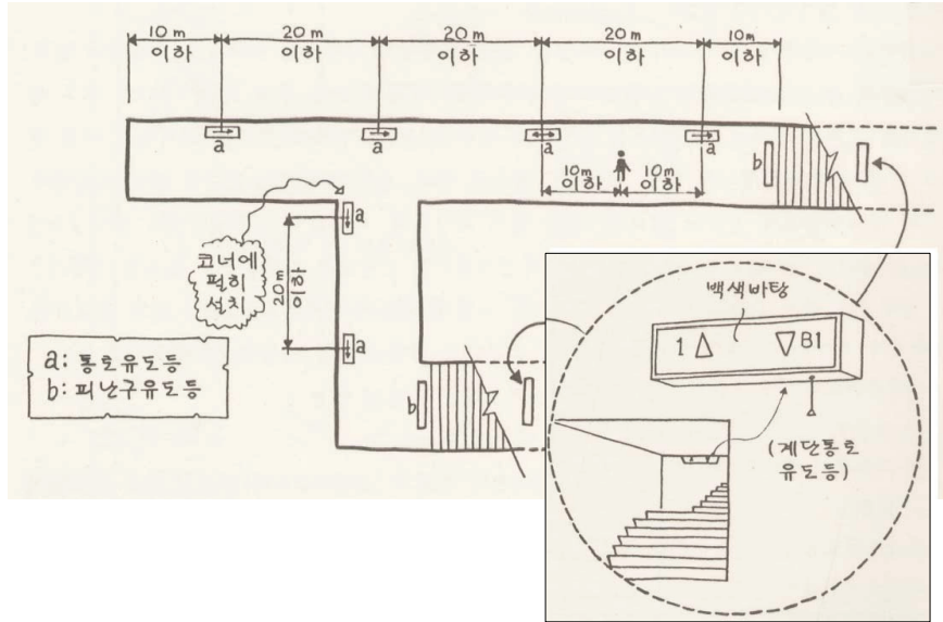
(그림 4) 통로유도등 및 피난구유도등의 설치기준
