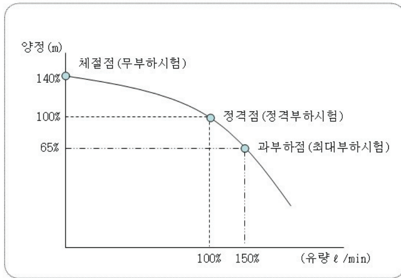
[소방펌프의 특성곡선]
