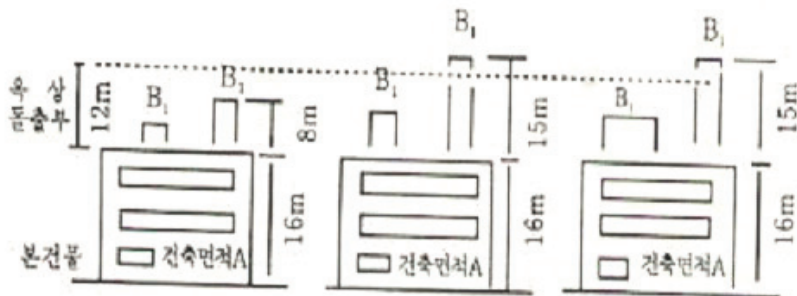
[그림 15] 옥상부분의 면적에 따른 건축물의 높이 산정
