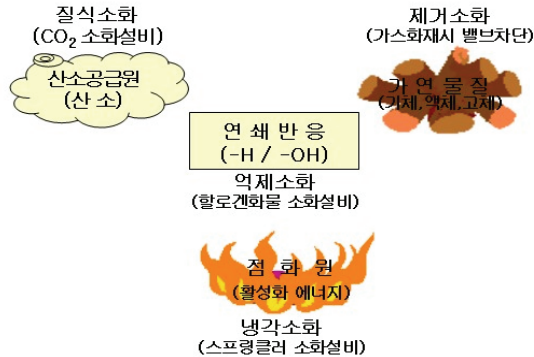
(그림1-1) 연소의 3요소 및 소화원리
