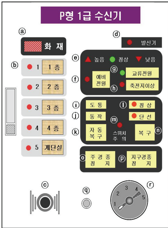
[그림 50] P형1급 수신기의 표시등 및 스위치
