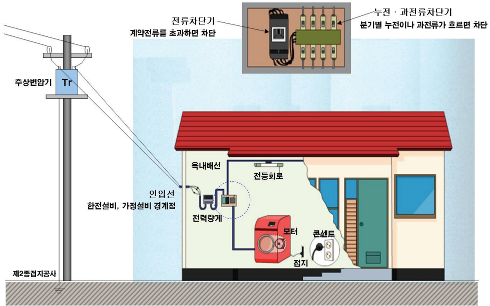
(그림 1) 일반주택의 옥내·외 배선
