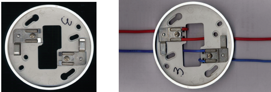
(그림 8) 감지기 베이스 및 배선방법
