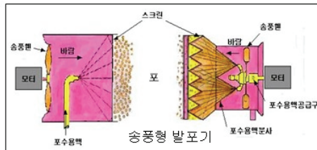
(그림 5-20) 흡출형/송풍형 고발포기
