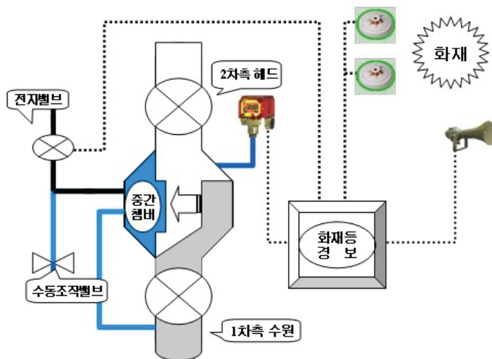
(그림 4-6) 준비작동식밸브 교차회로방식
