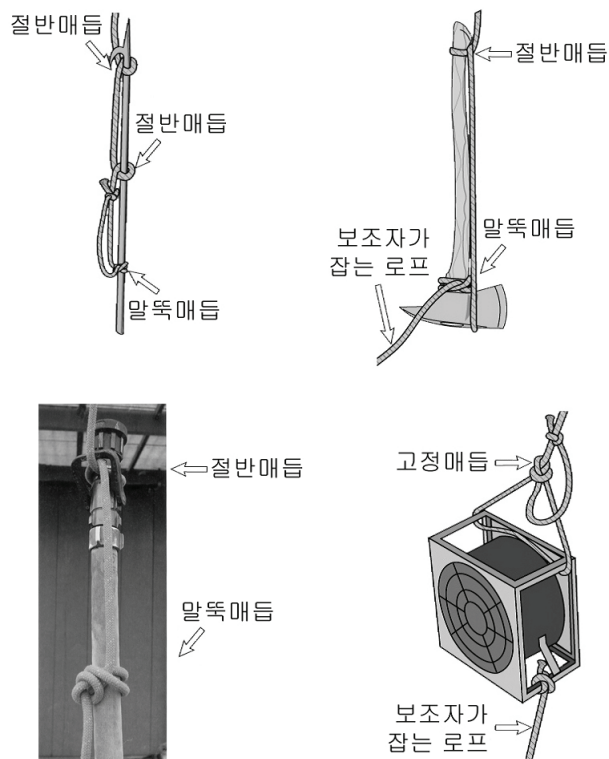
[그림 3-29] 여러가지 기구 묶기
