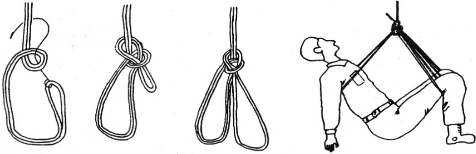
[그림 3-27] 세점고정매듭을 이용한 구조
