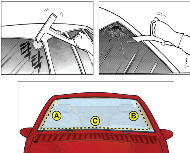
(그림 5-27) 앞 유리는 A,B 지점을 타격한 후 U자 형태로 잘라낸다.
