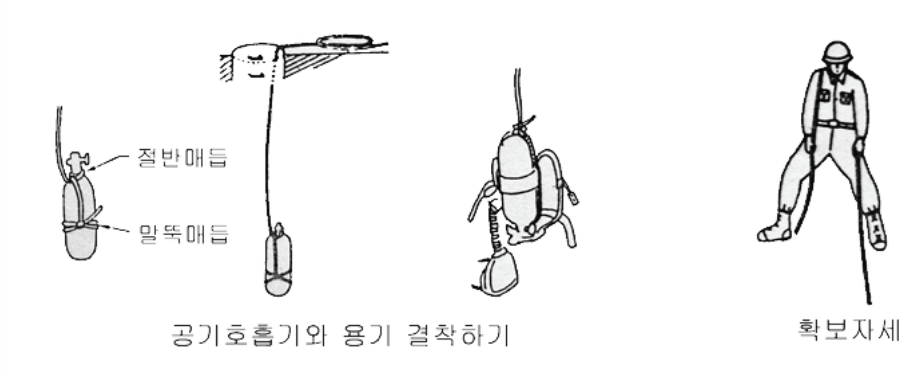
[그림 4-36] 폐쇄공간 진입법
