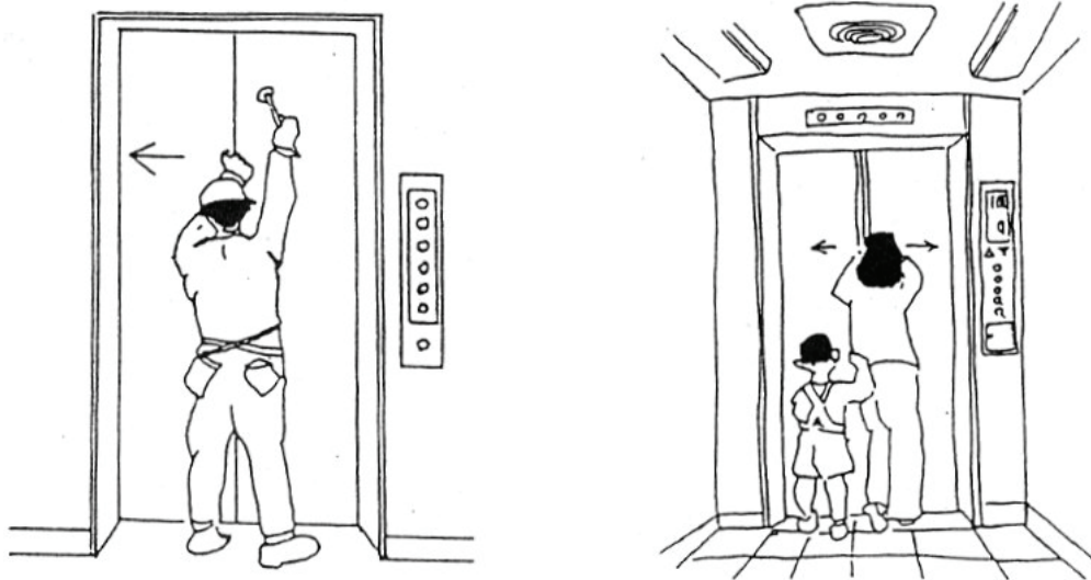
마스터키를 이용한 1차 문 개방(좌)
