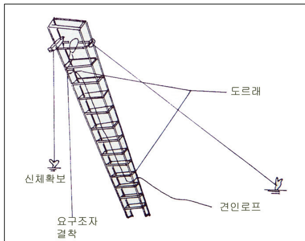
[그림 4-24] 인양구출 로프 설치방법
