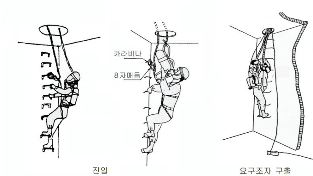
(그림 4-37) 폐쇄공간에서 요구조자 구출방법
