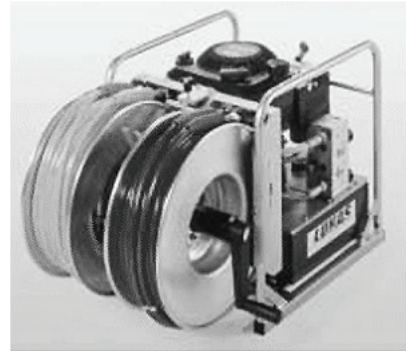
(그림 2-10) 호스릴이 부착된 유압엔진펌프
