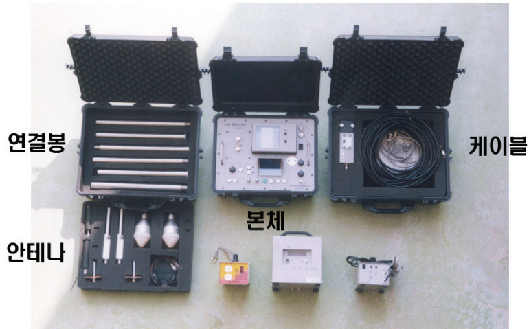
〔그림 2-20〕 매몰자전파탐지기
