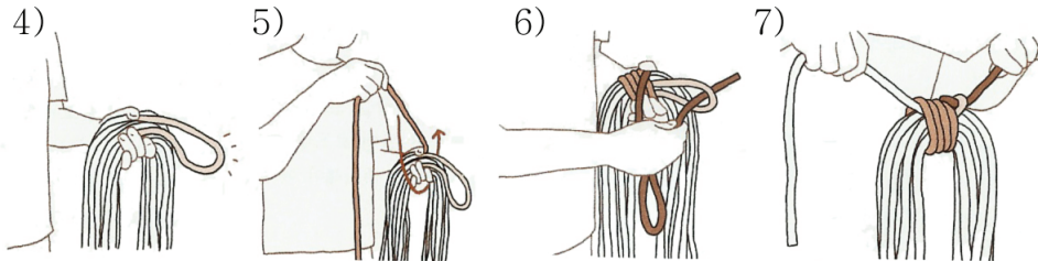
[그림 3-33] 로프 끝 가닥을 접어 고리를 만들고 다른 쪽 끝을 사려진 로프에 감은 후 끝을 고리에 통과시켜 당기고 마무리한다.
