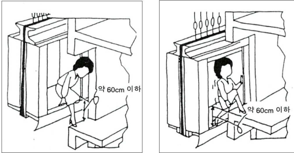
(그림 5-102) 승객의 구출 승장과 카의 높이 차이가 60cm 미만인 경우에는 승객이 직접 탈출할 수 있다.
