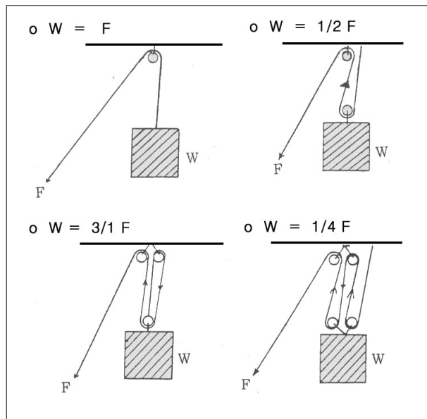
[그림 2-28] 도르래 숫자와 힘의 이득 관계
