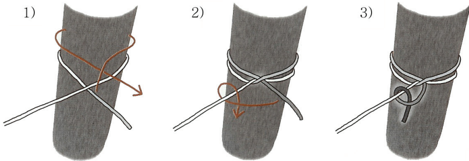
[그림 3-19] 말뚝매기의 로프 끝 처리법. 두 번 이상 절반매듭을 한다.
