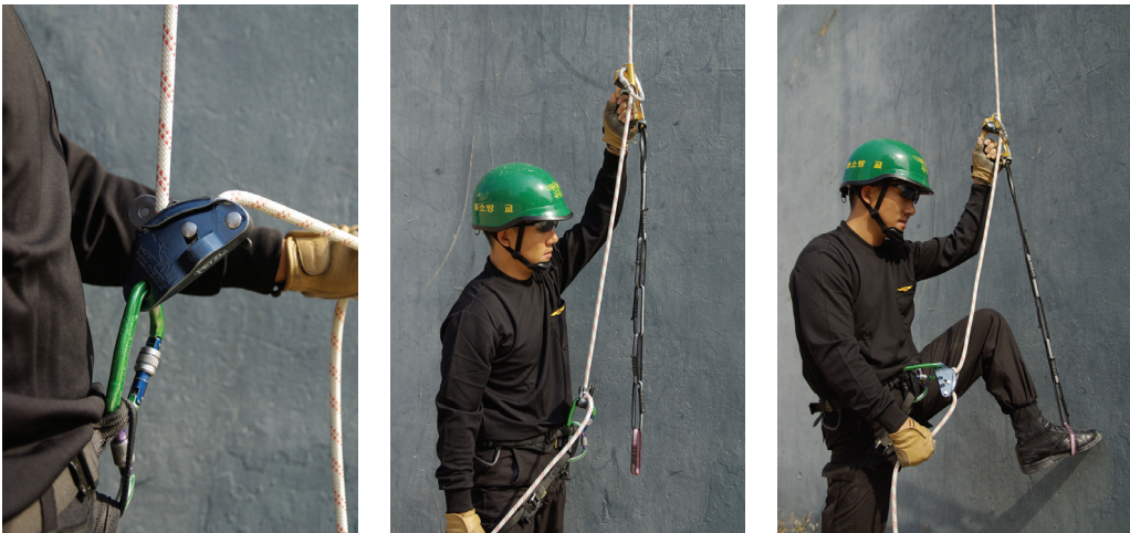
(그림 3-86) 그리그리와 쥘마에 현수로프를 삽입한다. 슬링의 고리에 발을 넣고 힘차게 일어선다.
