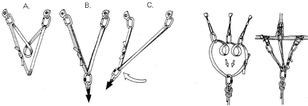
[그림 5-119] 확보물에 카라비나 걸기
