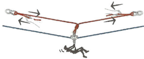
(그림 3-95) 다른 사람의 도움을 받아 이동하는 방법
