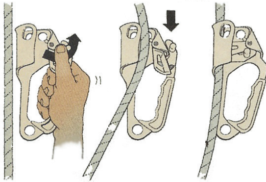
[그림 2-26] 등반기를 로프에 삽입하는 방법
